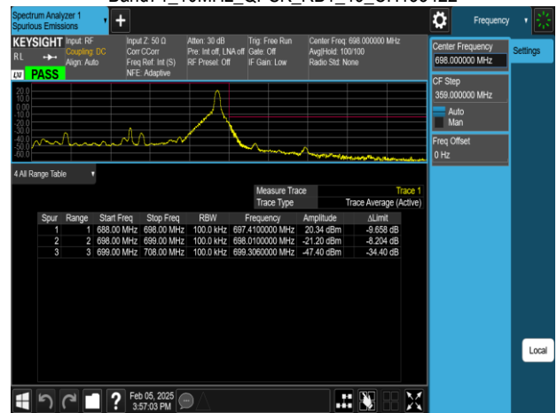
Band71_10MHz_QPSK_RB50_0_CH133422
