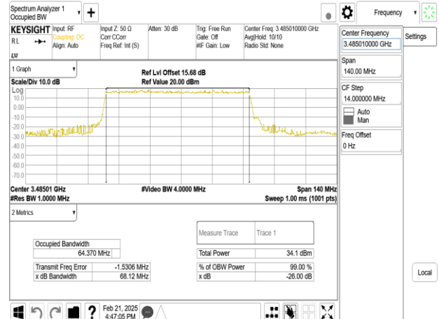
Band77-Part27_70MHz_DFT_s_OFDM_SCS30kHz_BPSK_RB180_0_CH632334
