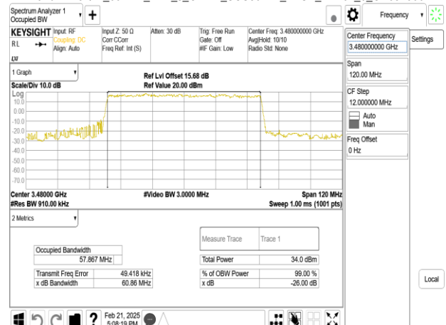
Band77-Part27_60MHz_DFT_s_OFDM_SCS30kHz_BPSK_RB162_0_CH632000
