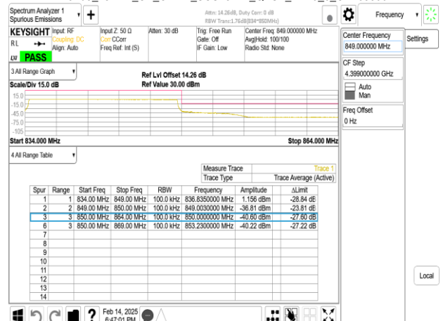
Band5_15MHz_CP_OFDM_SCS15kHz_QPSK_RB79_0_CH168300
