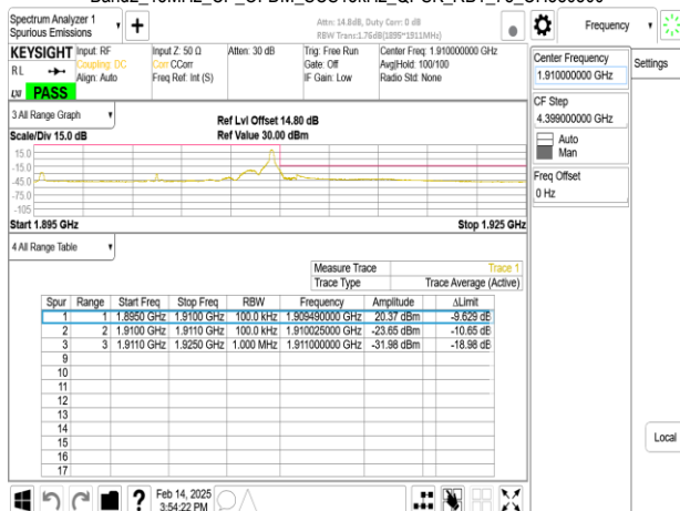
Band2_15MHz_CP_OFDM_SCS15kHz_QPSK_RB1_78_CH380500
