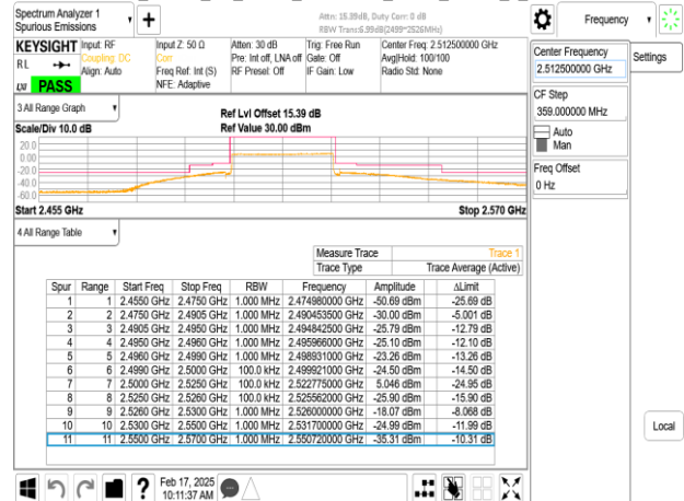
Band7_25MHz_CP_OFDM_SCS15kHz_QPSK_RB1_0_CH502500
