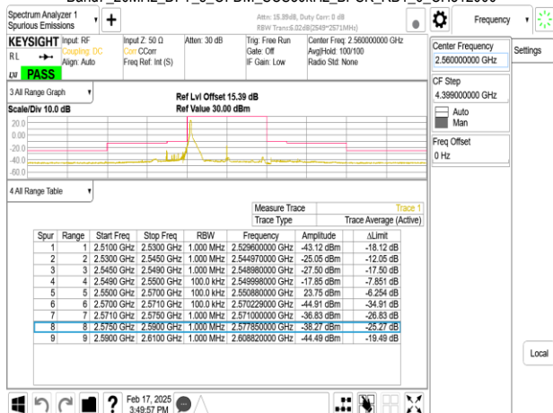
Band7_20MHz_DFT_s_OFDM_SCS30kHz_BPSK_RB1_50_CH512000
