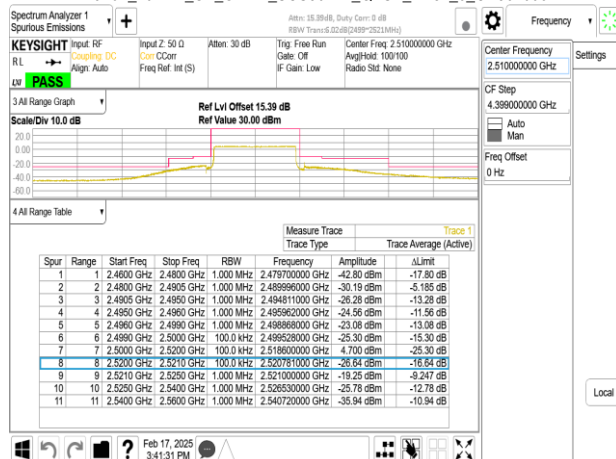
Band7_20MHz_CP_OFDM_SCS30kHz_QPSK_RB50_0_CH502000
