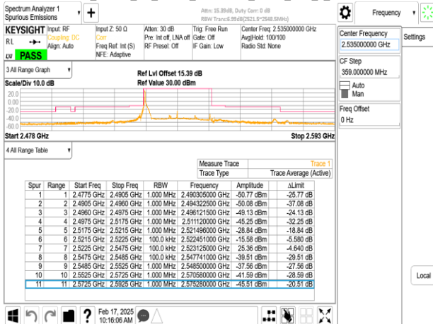
Band7_25MHz_CP_OFDM_SCS15kHz_QPSK_RB1_132_CH507000
