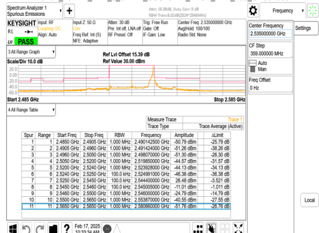
Band7_20MHz_DFT_s_OFDM_SCS15kHz_BPSK_RB1_105_CH507000
