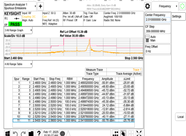
Band7_20MHz_CP_OFDM_SCS15kHz_QPSK_RB1_105_CH502000
