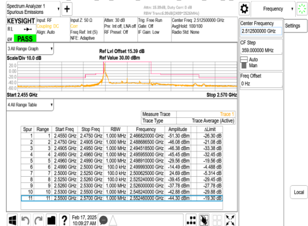
Band7_25MHz_CP_OFDM_SCS15kHz_QPSK_RB1_132_CH502500
