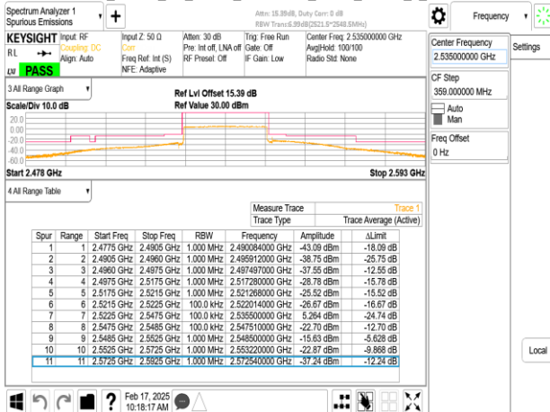
Band7_25MHz_CP_OFDM_SCS15kHz_QPSK_RB1_0_CH507000
