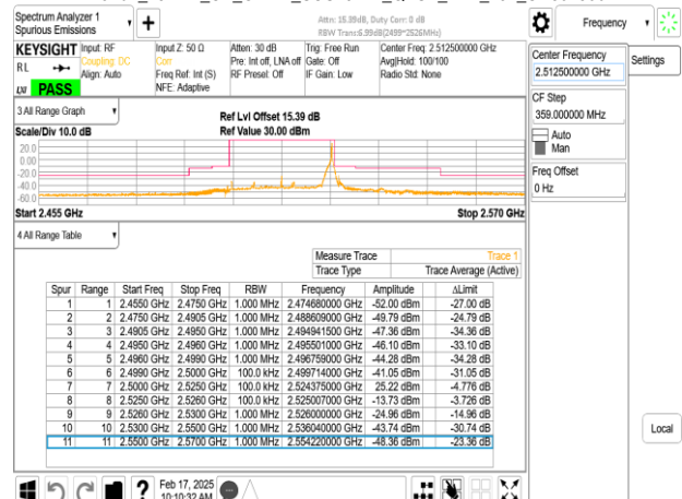
Band7_25MHz_CP_OFDM_SCS15kHz_QPSK_RB1_132_CH502500
