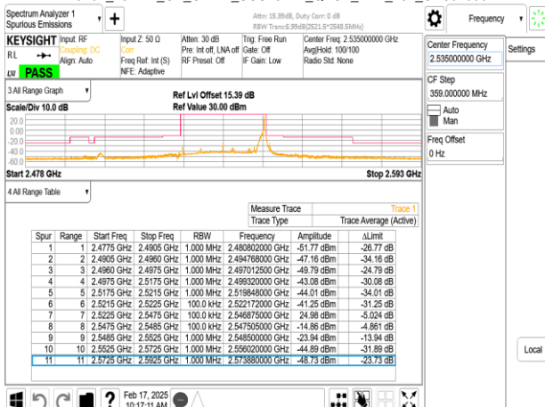
Band7_25MHz_CP_OFDM_SCS15kHz_QPSK_RB1_132_CH507000
