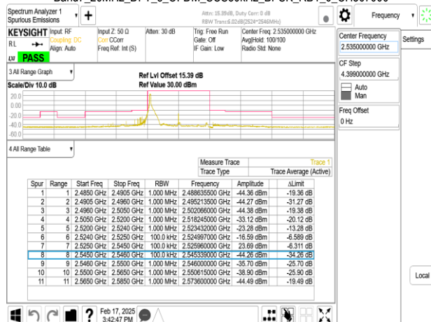
Band7_20MHz_DFT_s_OFDM_SCS30kHz_BPSK_RB1_50_CH507000
