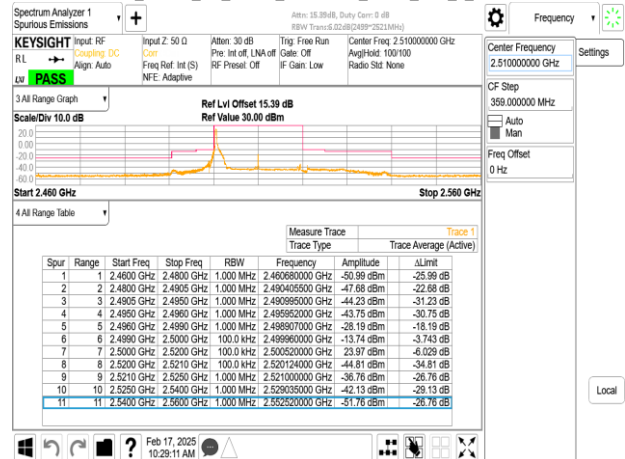
Band7_20MHz_CP_OFDM_SCS15kHz_QPSK_RB1_105_CH502000
