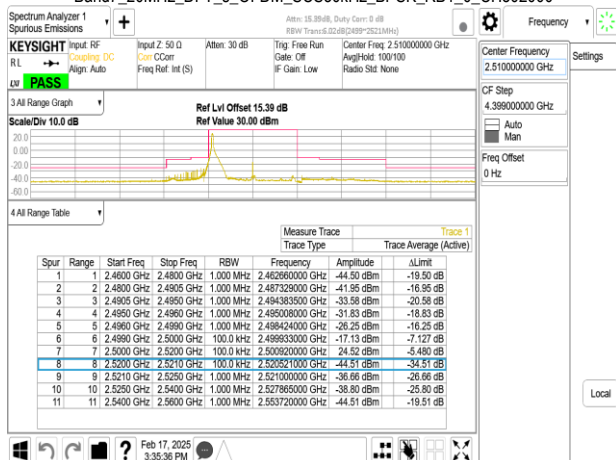
Band7_20MHz_DFT_s_OFDM_SCS30kHz_BPSK_RB1_50_CH502000
