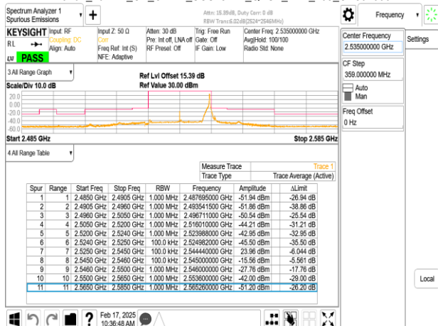
Band7_20MHz_CP_OFDM_SCS15kHz_QPSK_RB1_105_CH507000
