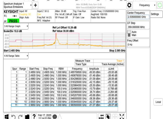
Band7_20MHz_DFT_s_OFDM_SCS15kHz_BPSK_RB1_105_CH507000
