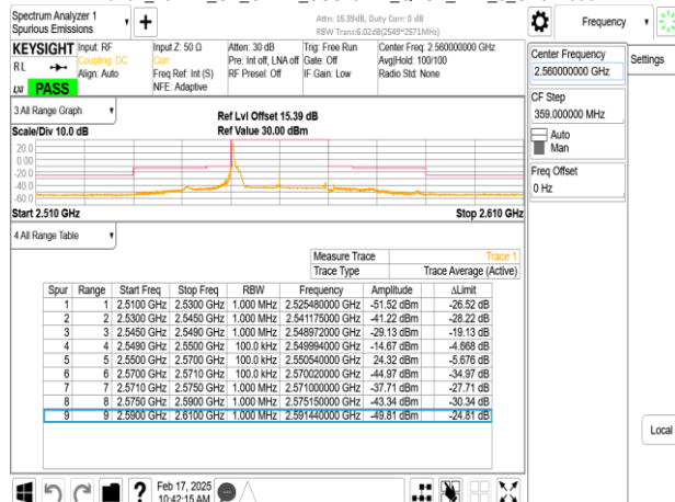
Band7_20MHz_CP_OFDM_SCS15kHz_QPSK_RB1_105_CH512000
