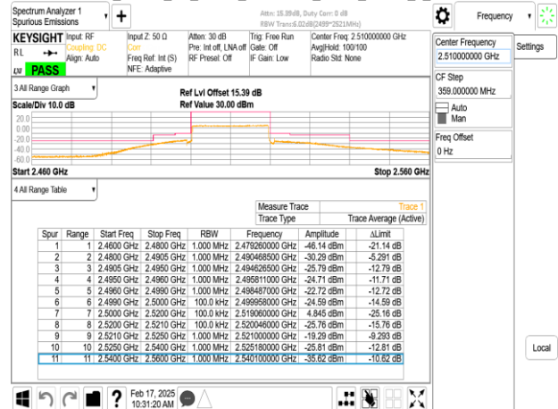
Band7_20MHz_CP_OFDM_SCS15kHz_QPSK_RB1_0_CH502000
