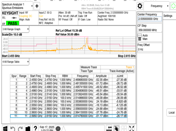
Band7_40MHz_CP_OFDM_SCS30kHz_QPSK_RB1_105_CH507000
