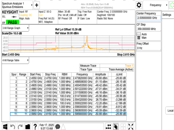
Band7_40MHz_CP_OFDM_SCS15kHz_QPSK_RB216_0_CH507000
