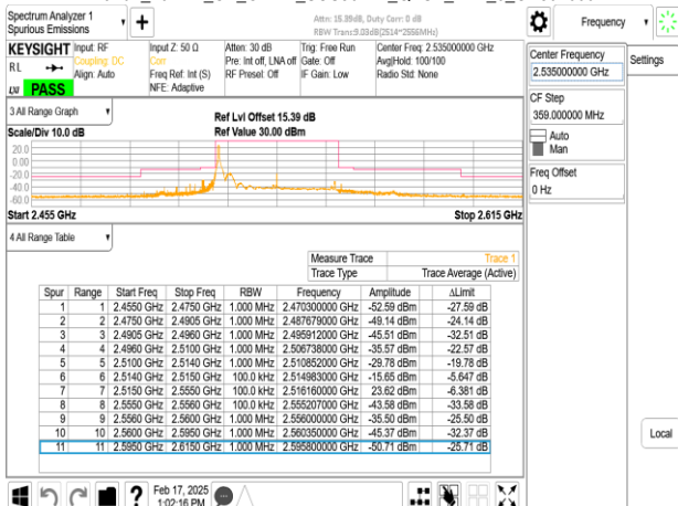
Band7_40MHz_CP_OFDM_SCS30kHz_QPSK_RB1_105_CH507000
