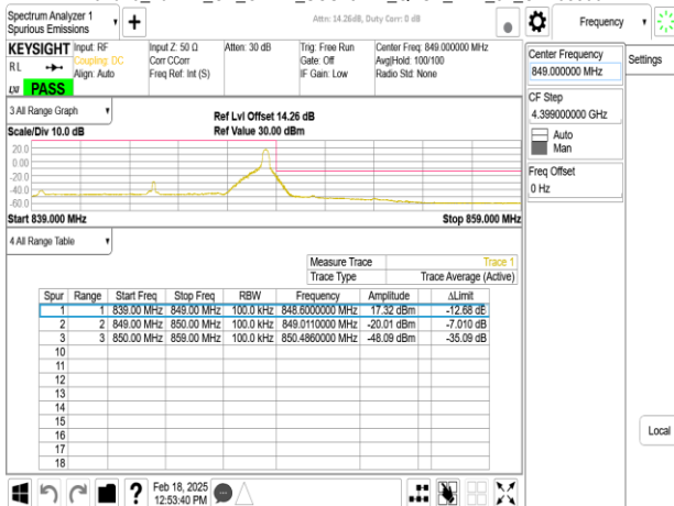
Band26_10MHz_CP_OFDM_SCS15kHz_QPSK_RB52_0_CH168800
