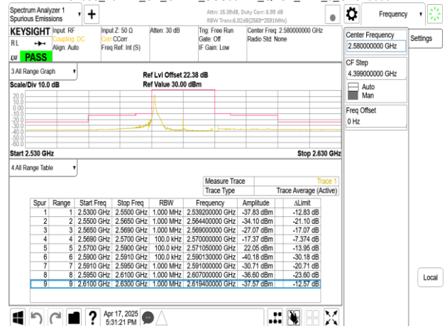
Band38_20MHz_CP_OFDM_SCS30kHz_QPSK_RB1_50_CH516000
