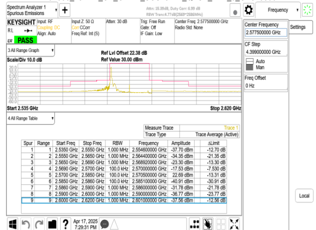
Band38_15MHz_CP_OFDM_SCS15kHz_QPSK_RB1_78_CH515500
