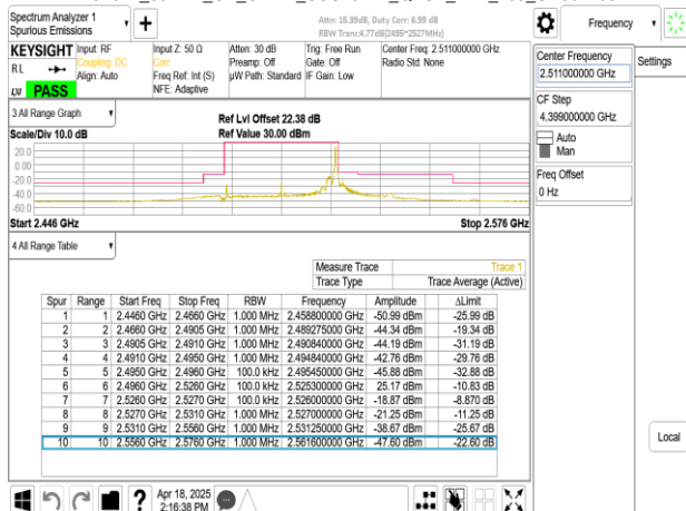
Band41_30MHz_CP_OFDM_SCS15kHz_QPSK_RB1_159_CH502200
