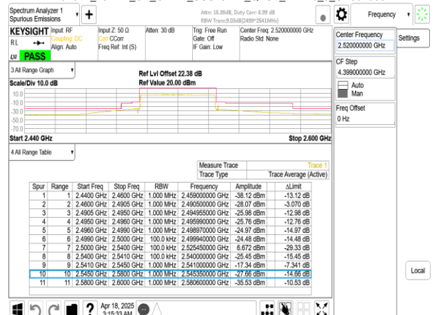
Band41_40MHz_CP_OFDM_SCS15kHz_QPSK_RB216_0_CH504000
