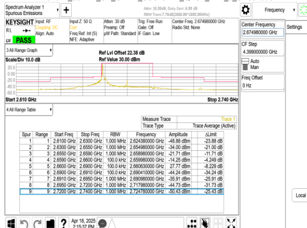
Band41_30MHz_CP_OFDM_SCS15kHz_QPSK_RB1_159_CH534996
