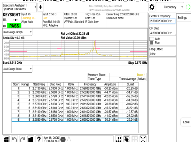
Band41_40MHz_CP_OFDM_SCS30kHz_QPSK_RB1_105_CH518604
