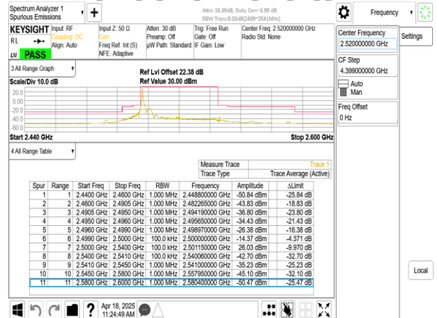
Band41_40MHz_CP_OFDM_SCS30kHz_QPSK_RB1_105_CH504000
