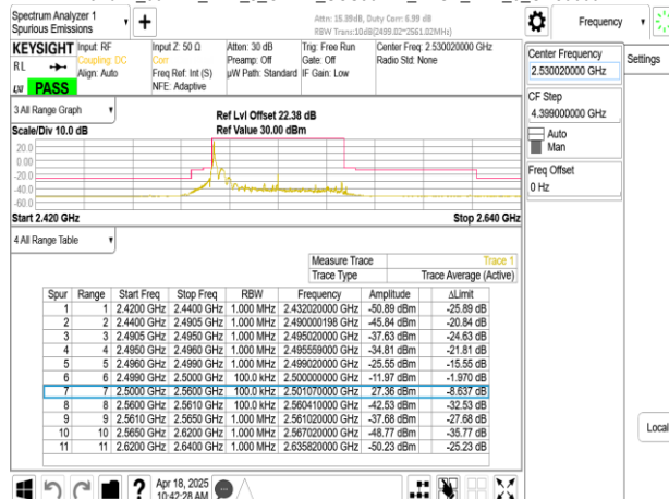
Band41_60MHz_DFT_s_OFDM_SCS30kHz_BPSK_RB1_161_CH506004
