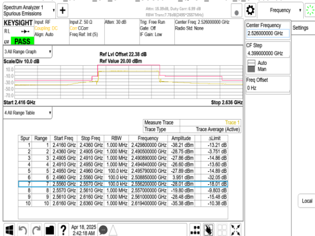
Band41_60MHz_CP_OFDM_SCS30kHz_QPSK_RB1_0_CH505200
