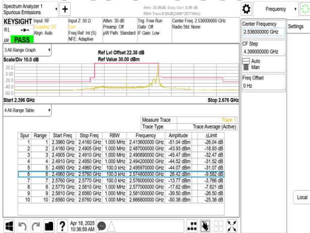
Band41_80MHz_CP_OFDM_SCS30kHz_QPSK_RB217_0_CH507204
