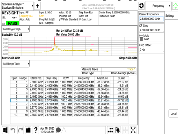
Band41_80MHz_CP_OFDM_SCS30kHz_QPSK_RB1_216_CH507204
