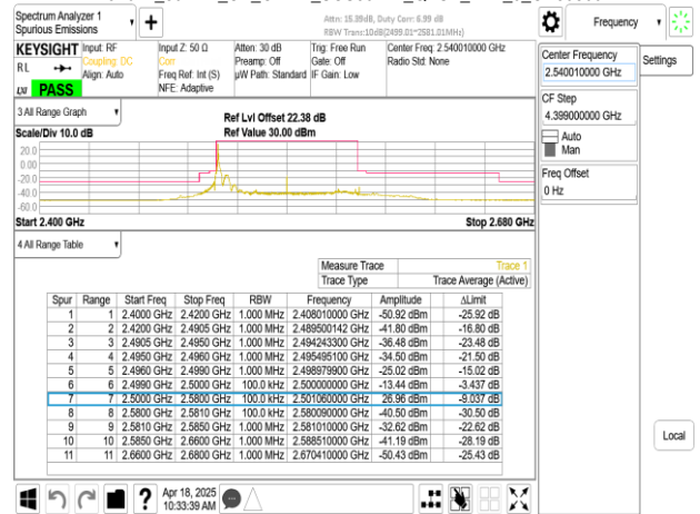
Band41_80MHz_CP_OFDM_SCS30kHz_QPSK_RB1_216_CH508002
