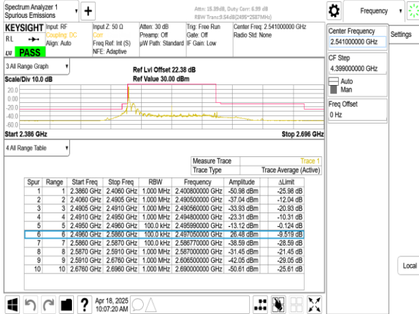
Band41_90MHz_CP_OFDM_SCS30kHz_QPSK_RB1_244_CH508200
