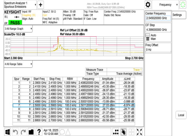
Band41_90MHz_CP_OFDM_SCS30kHz_QPSK_RB1_244_CH509004
