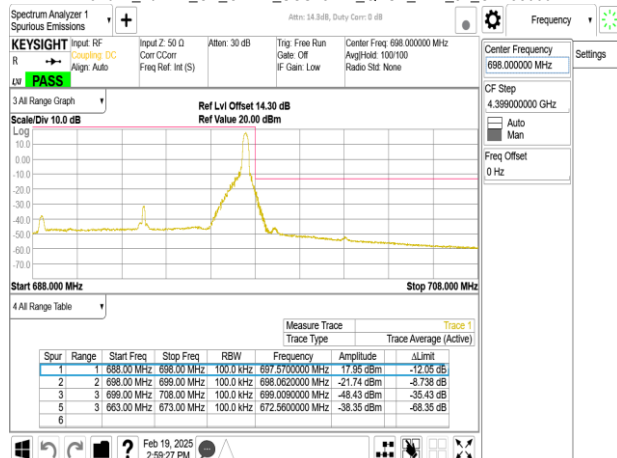
Band71_10MHz_CP_OFDM_SCS15kHz_QPSK_RB52_0_CH138600
