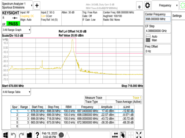
Band71_20MHz_CP_OFDM_SCS30kHz_QPSK_RB1_50_CH137600
