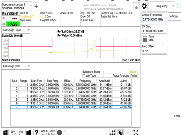
Band77-Part27_15MHz_CP_OFDM_SCS15kHz_QPSK_RB1_78_CH664832
