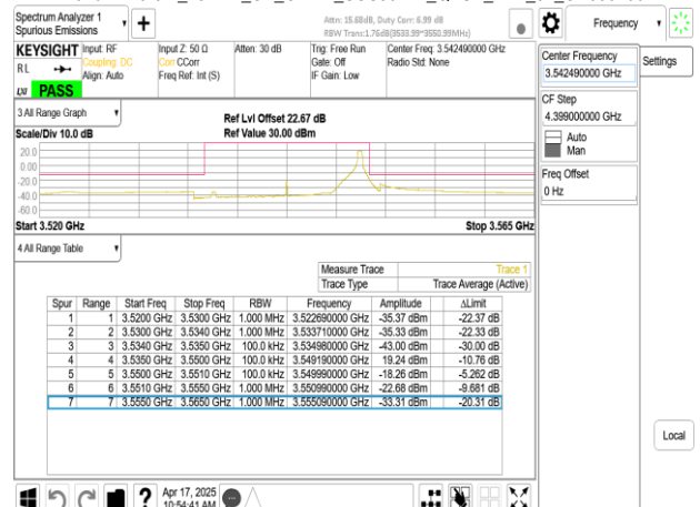
Band77-Part27_15MHz_CP_OFDM_SCS30kHz_QPSK_RB1_37_CH636166
