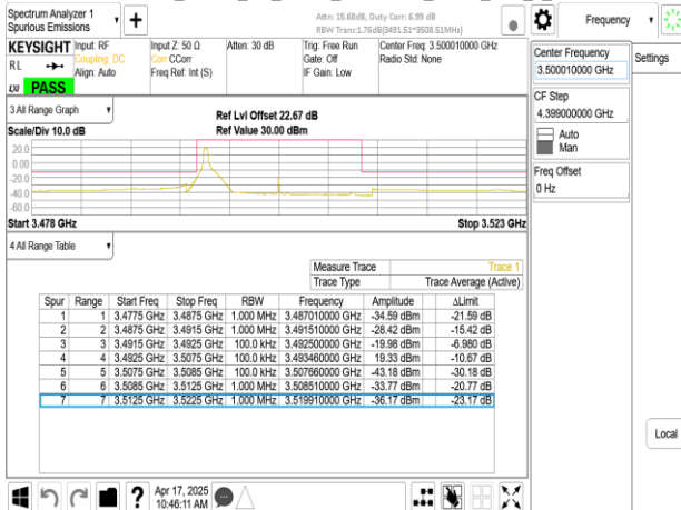
Band77-Part27_15MHz_CP_OFDM_SCS30kHz_QPSK_RB1_37_CH633334
