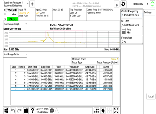
Band77-Part27_15MHz_CP_OFDM_SCS30kHz_QPSK_RB1_37_CH630500
