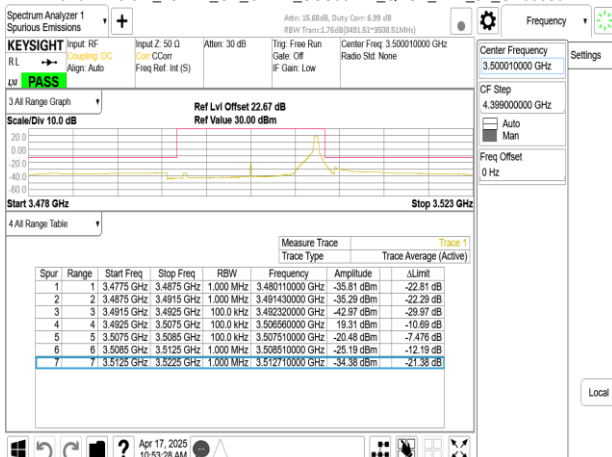
Band77-Part27_15MHz_CP_OFDM_SCS30kHz_QPSK_RB1_37_CH633334
