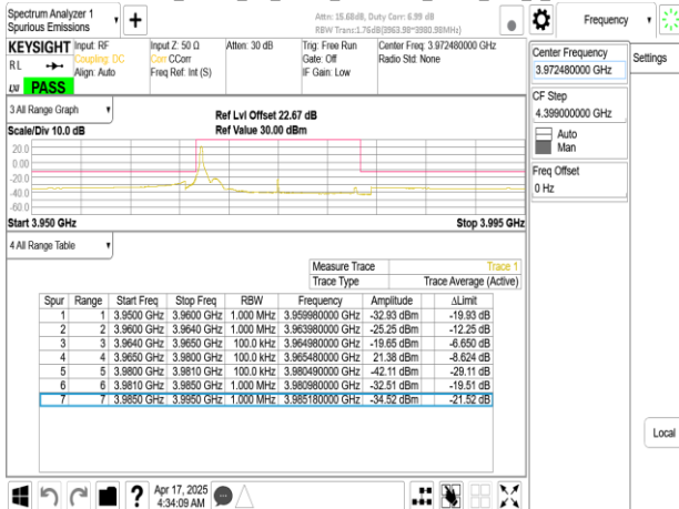
Band77-Part27_15MHz_CP_OFDM_SCS15kHz_QPSK_RB1_78_CH664832
