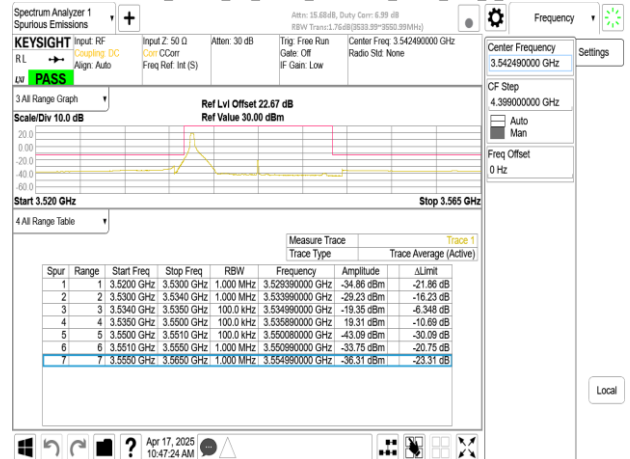
Band77-Part27_15MHz_CP_OFDM_SCS30kHz_QPSK_RB1_37_CH636166
