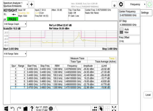
Band77-Part27_15MHz_CP_OFDM_SCS30kHz_QPSK_RB1_37_CH630500
