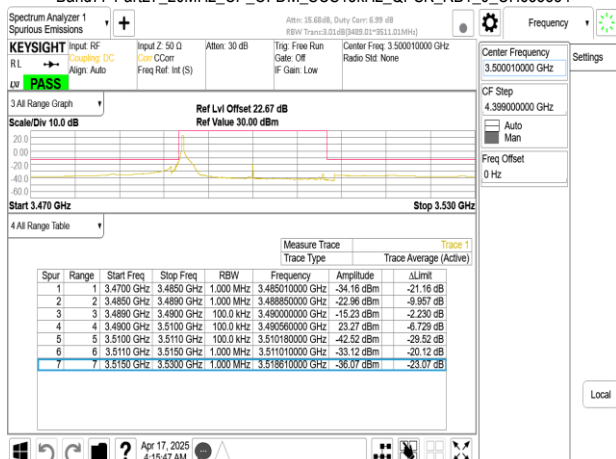
Band77-Part27_20MHz_CP_OFDM_SCS15kHz_QPSK_RB1_0_CH633334
