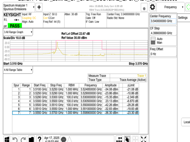
Band77-Part27_20MHz_CP_OFDM_SCS15kHz_QPSK_RB1_0_CH636000
