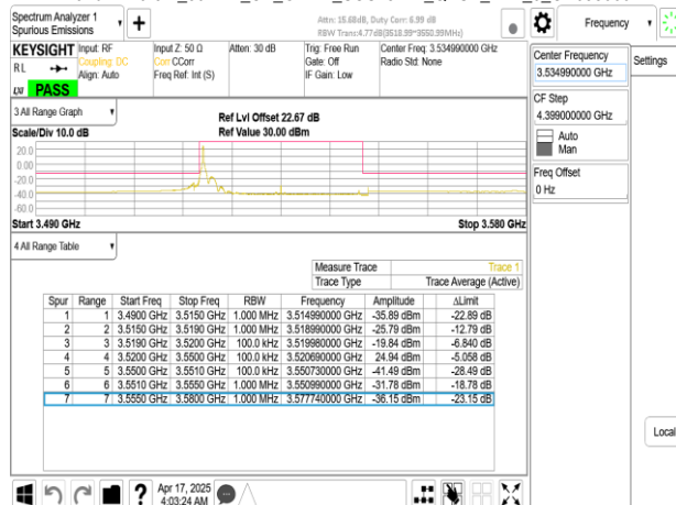
Band77-Part27_30MHz_CP_OFDM_SCS15kHz_QPSK_RB1_0_CH635666
