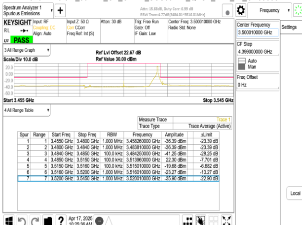
Band77-Part27_30MHz_CP_OFDM_SCS30kHz_QPSK_RB1_77_CH633334
