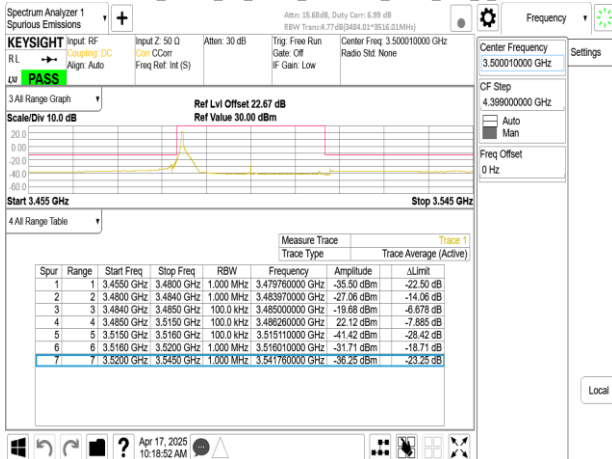
Band77-Part27_30MHz_CP_OFDM_SCS30kHz_QPSK_RB1_77_CH633334
