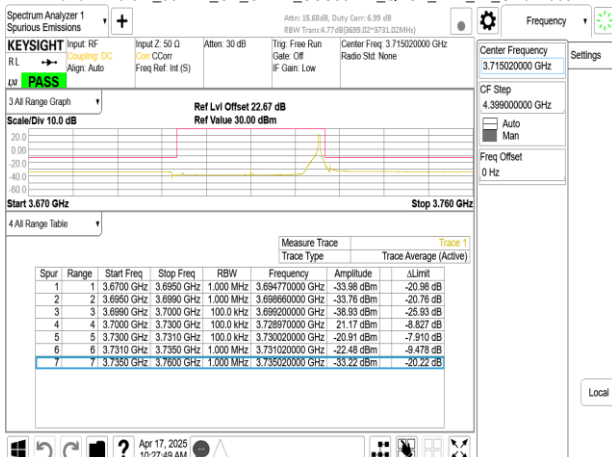
Band77-Part27_30MHz_CP_OFDM_SCS30kHz_QPSK_RB1_77_CH647668
