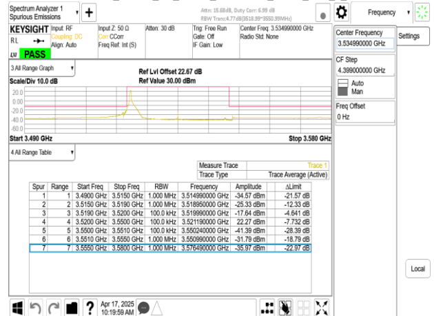
Band77-Part27_30MHz_CP_OFDM_SCS30kHz_QPSK_RB1_77_CH635666
