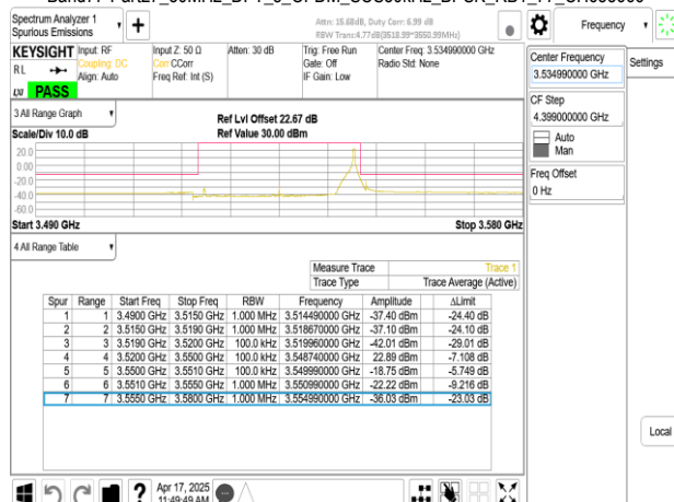
Band77-Part27_30MHz_DFT_s_OFDM_SCS30kHz_BPSK_RB1_77_CH635666
