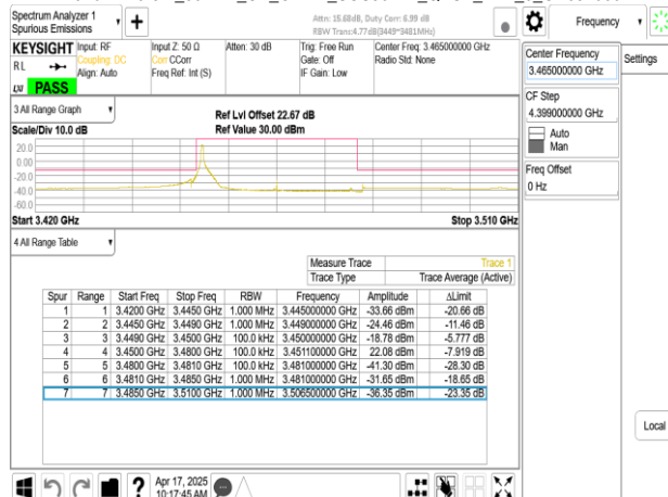
Band77-Part27_30MHz_CP_OFDM_SCS30kHz_QPSK_RB1_77_CH631000
