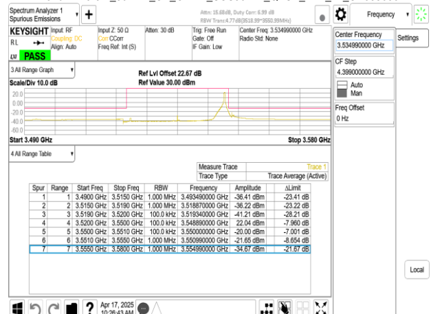
Band77-Part27_30MHz_CP_OFDM_SCS30kHz_QPSK_RB1_77_CH635666
