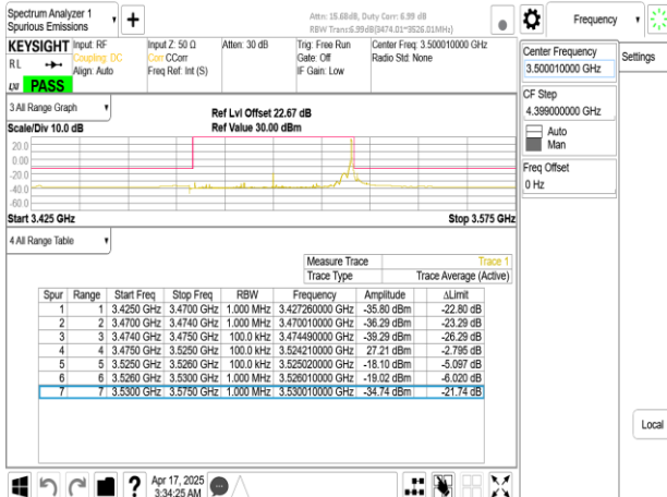
Band77-Part27_50MHz_CP_OFDM_SCS15kHz_QPSK_RB1_269_CH633334
