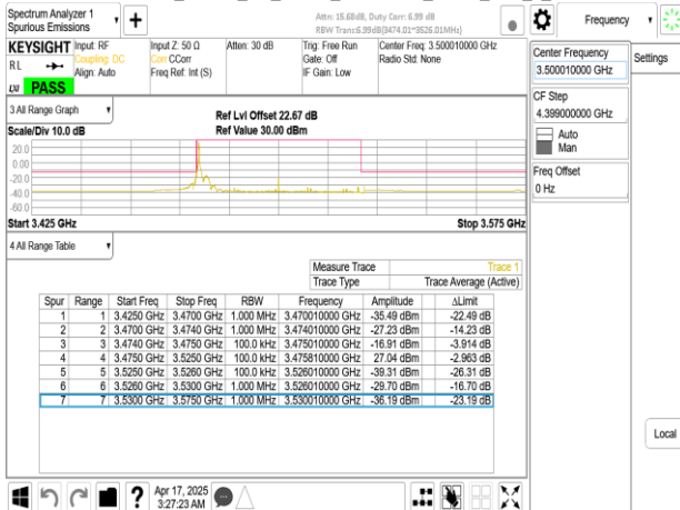
Band77-Part27_50MHz_CP_OFDM_SCS15kHz_QPSK_RB1_269_CH633334
