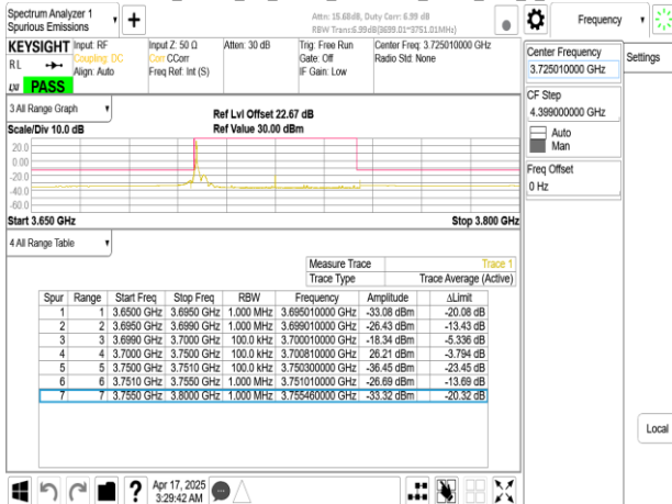
Band77-Part27_50MHz_CP_OFDM_SCS15kHz_QPSK_RB1_269_CH648334
