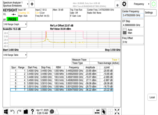
Band77-Part27_50MHz_CP_OFDM_SCS15kHz_QPSK_RB1_269_CH631668
