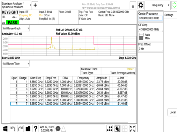
Band77-Part27_50MHz_CP_OFDM_SCS15kHz_QPSK_RB1_269_CH663666
