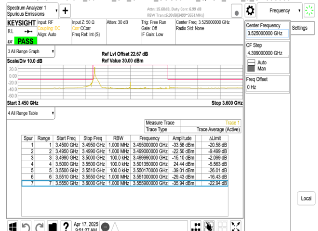
Band77-Part27_50MHz_CP_OFDM_SCS30kHz_QPSK_RB1_0_CH635000
