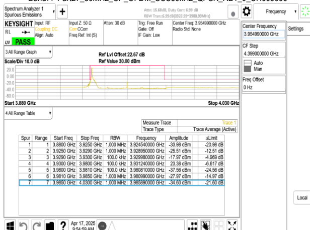
Band77-Part27_50MHz_CP_OFDM_SCS30kHz_QPSK_RB1_0_CH663666
