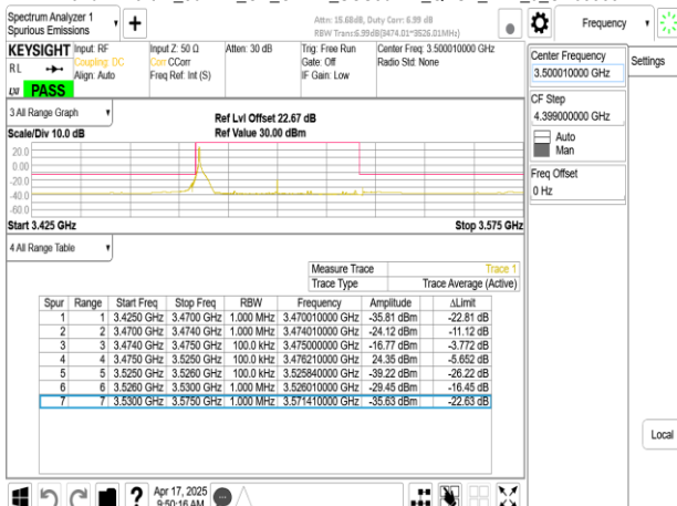
Band77-Part27_50MHz_CP_OFDM_SCS30kHz_QPSK_RB1_0_CH633334
