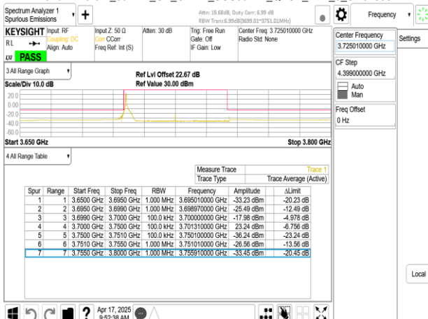
Band77-Part27_50MHz_CP_OFDM_SCS30kHz_QPSK_RB1_0_CH648334
