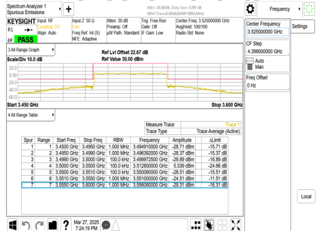
Band77-Part27_50MHz_CP_OFDM_SCS30kHz_QPSK_RB1_0_CH635000
