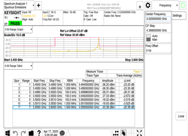
Band77-Part27_50MHz_CP_OFDM_SCS15kHz_QPSK_RB1_269_CH635000
