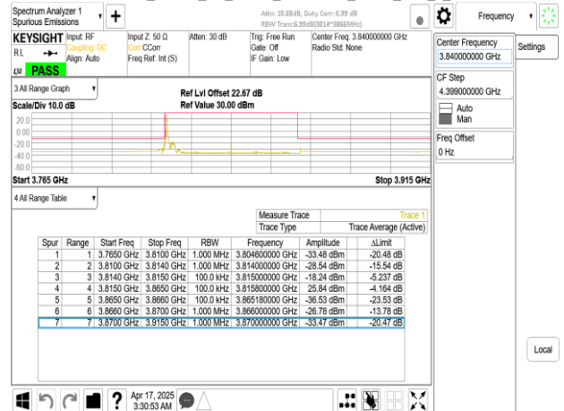
Band77-Part27_50MHz_CP_OFDM_SCS15kHz_QPSK_RB1_269_CH656000
