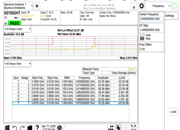
Band77-Part27_50MHz_CP_OFDM_SCS15kHz_QPSK_RB1_269_CH656000
