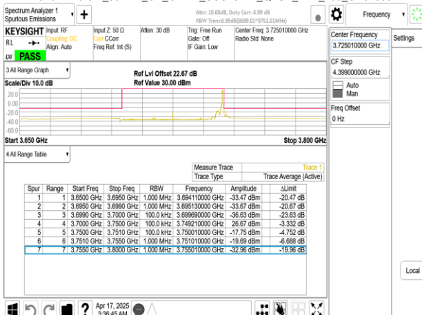
Band77-Part27_50MHz_CP_OFDM_SCS15kHz_QPSK_RB1_269_CH648334
