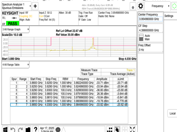
Band77-Part27_50MHz_CP_OFDM_SCS15kHz_QPSK_RB1_269_CH663666
