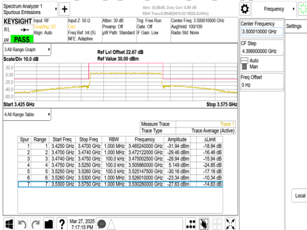
Band77-Part27_50MHz_CP_OFDM_SCS30kHz_QPSK_RB1_0_CH633334
