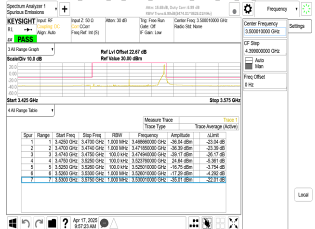
Band77-Part27_50MHz_CP_OFDM_SCS30kHz_QPSK_RB133_0_CH635000
