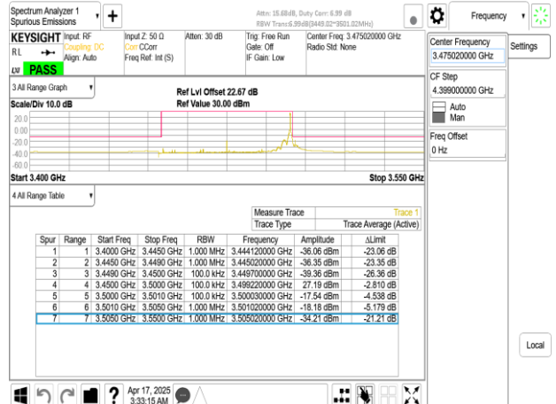
Band77-Part27_50MHz_CP_OFDM_SCS15kHz_QPSK_RB1_269_CH631668
