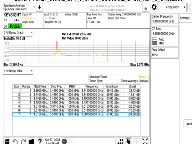
Band77-Part27_60MHz_DFT_s_OFDM_SCS30kHz_BPSK_RB1_0_CH632000
