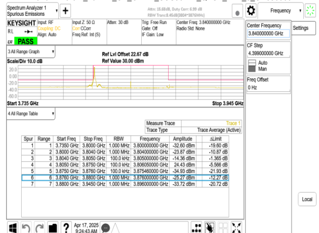
Band77-Part27_70MHz_CP_OFDM_SCS30kHz_QPSK_RB1_0_CH656000
