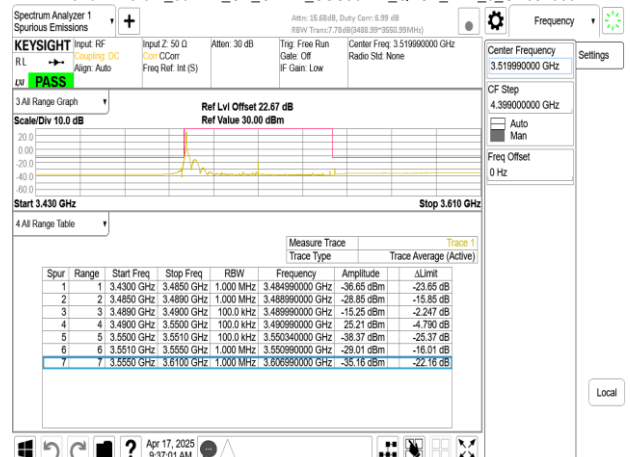
Band77-Part27_60MHz_CP_OFDM_SCS30kHz_QPSK_RB1_0_CH634666
