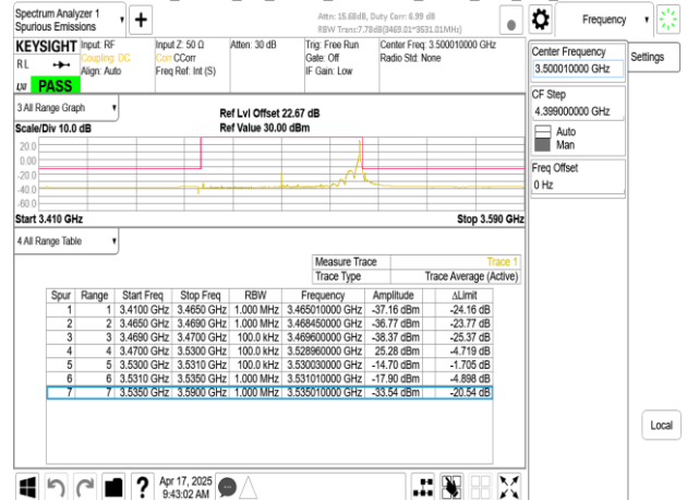
Band77-Part27_60MHz_CP_OFDM_SCS30kHz_QPSK_RB162_0_CH634666
