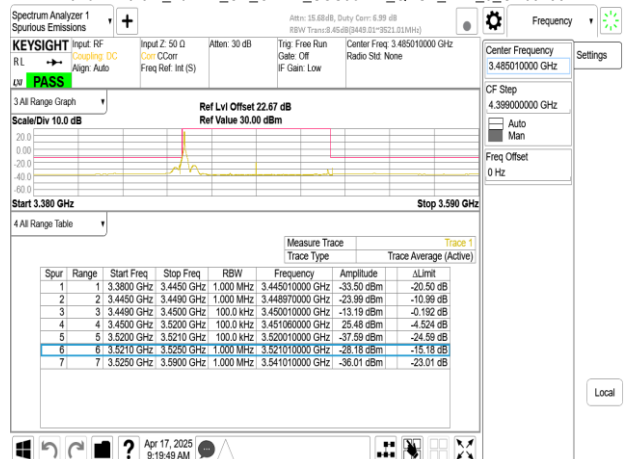
Band77-Part27_70MHz_CP_OFDM_SCS30kHz_QPSK_RB1_0_CH632334
