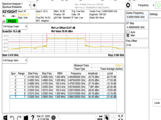
Band77-Part27_60MHz_DFT_s_OFDM_SCS30kHz_BPSK_RB1_0_CH633334
