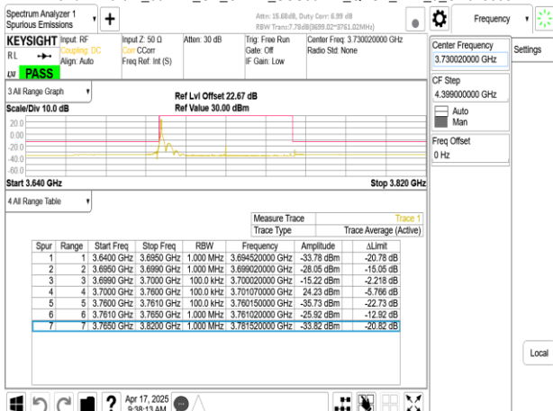
Band77-Part27_60MHz_CP_OFDM_SCS30kHz_QPSK_RB1_0_CH648668
