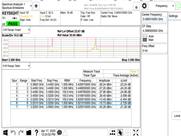
Band77-Part27_70MHz_DFT_s_OFDM_SCS30kHz_BPSK_RB180_0_CH633334
