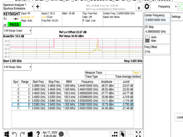
Band77-Part27_70MHz_CP_OFDM_SCS30kHz_QPSK_RB189_0_CH634332
