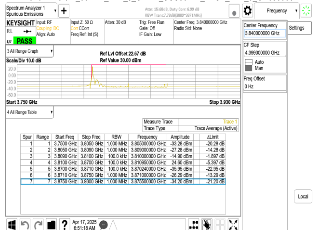
Band77-Part27_60MHz_DFT_s_OFDM_SCS30kHz_BPSK_RB1_0_CH656000
