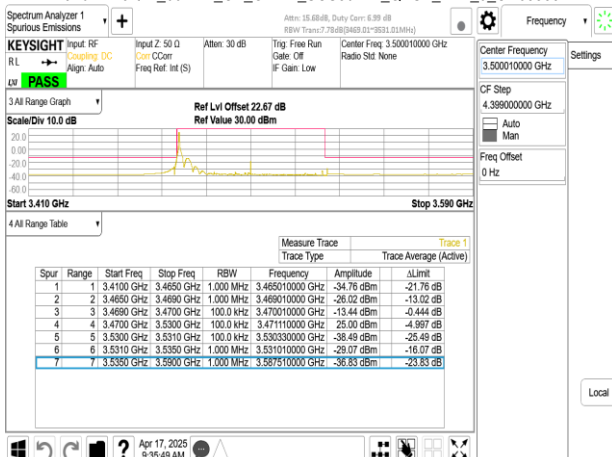
Band77-Part27_60MHz_CP_OFDM_SCS30kHz_QPSK_RB1_0_CH633334
