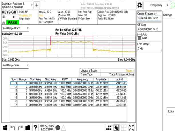
Band77-Part27_60MHz_CP_OFDM_SCS30kHz_QPSK_RB1_0_CH663332
