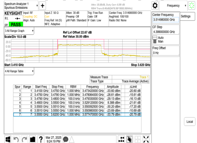
Band77-Part27_70MHz_DFT_s_OFDM_SCS30kHz_BPSK_RB1_0_CH634332
