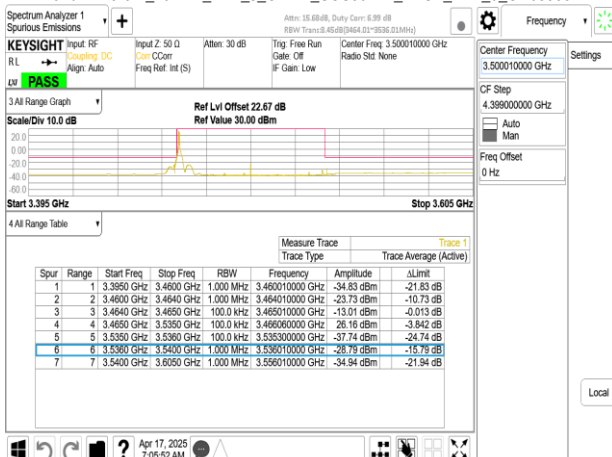
Band77-Part27_70MHz_DFT_s_OFDM_SCS30kHz_BPSK_RB1_0_CH633334
