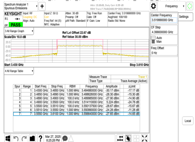
Band77-Part27_60MHz_CP_OFDM_SCS30kHz_QPSK_RB1_0_CH634666
