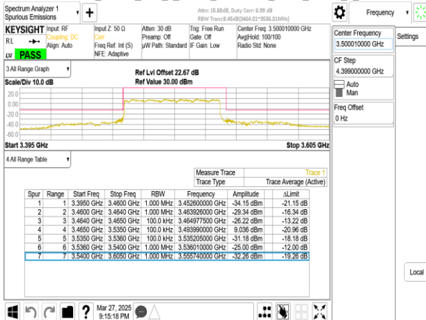
Band77-Part27_70MHz_DFT_s_OFDM_SCS30kHz_BPSK_RB1_0_CH633334
