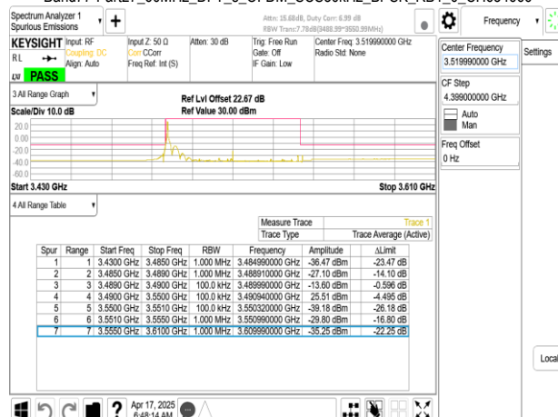
Band77-Part27_60MHz_DFT_s_OFDM_SCS30kHz_BPSK_RB1_0_CH634666
