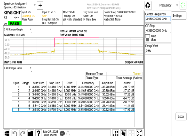
Band77-Part27_60MHz_CP_OFDM_SCS30kHz_QPSK_RB1_0_CH632000
