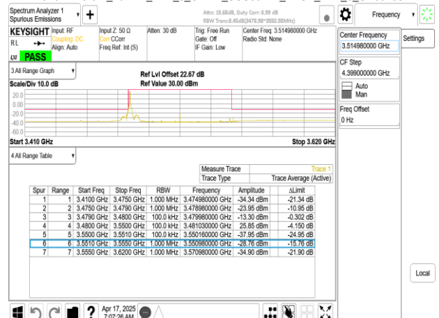
Band77-Part27_70MHz_DFT_s_OFDM_SCS30kHz_BPSK_RB1_0_CH634332
