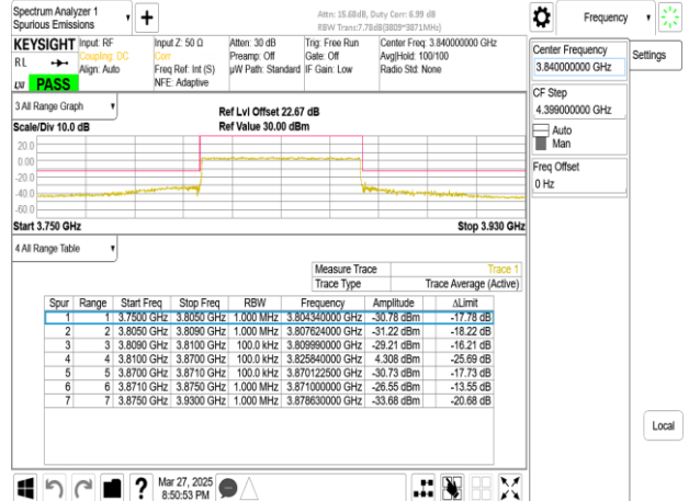
Band77-Part27_60MHz_CP_OFDM_SCS30kHz_QPSK_RB1_0_CH656000
