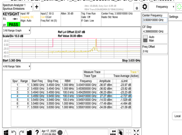
Band77-Part27_90MHz_DFT_s_OFDM_SCS30kHz_BPSK_RB1_244_CH633334
