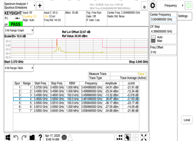
Band77-Part27_90MHz_CP_OFDM_SCS30kHz_QPSK_RB1_244_CH633666
