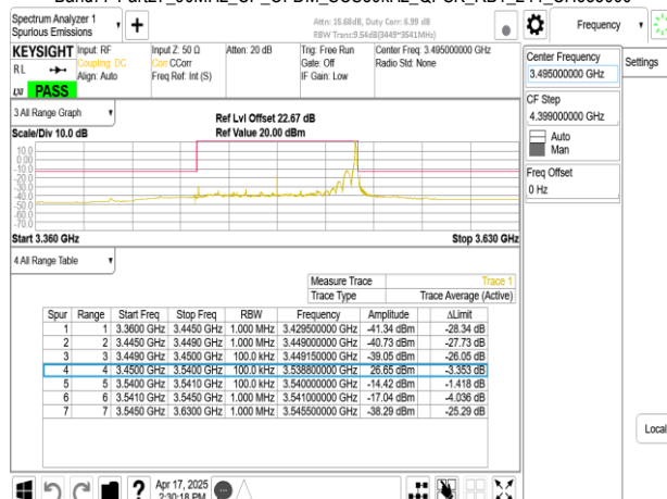
Band77-Part27_90MHz_CP_OFDM_SCS30kHz_QPSK_RB1_244_CH633000
