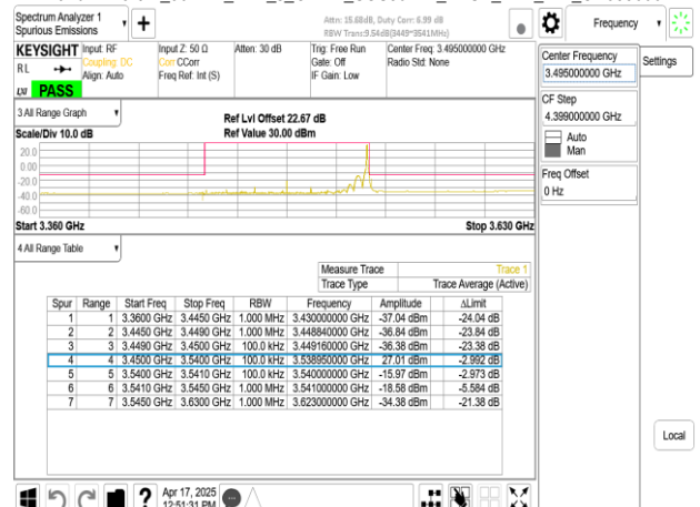
Band77-Part27_90MHz_DFT_s_OFDM_SCS30kHz_BPSK_RB1_244_CH633000
