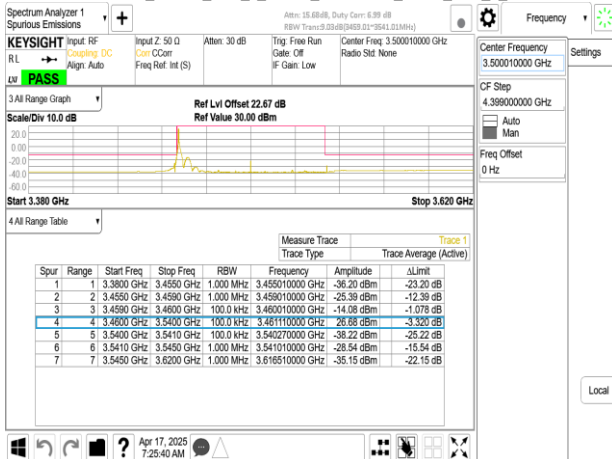
Band77-Part27_80MHz_DFT_s_OFDM_SCS30kHz_BPSK_RB1_216_CH633334
