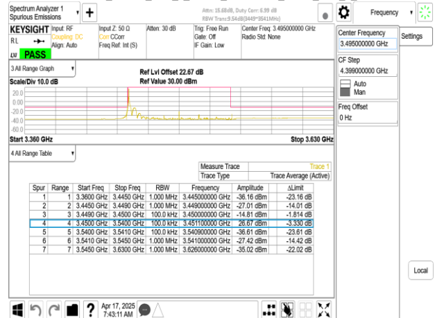
Band77-Part27_90MHz_DFT_s_OFDM_SCS30kHz_BPSK_RB1_244_CH633000
