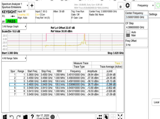
Band77-Part27_80MHz_DFT_s_OFDM_SCS30kHz_BPSK_RB1_216_CH633334
