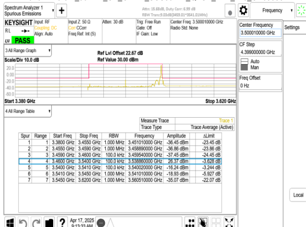
Band77-Part27_80MHz_CP_OFDM_SCS30kHz_QPSK_RB1_216_CH633334
