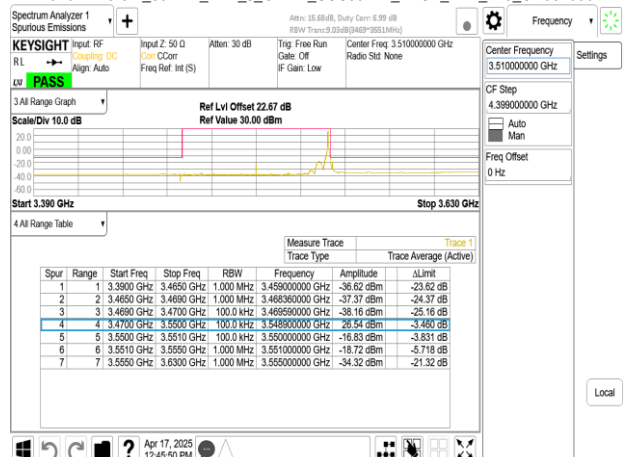
Band77-Part27_80MHz_DFT_s_OFDM_SCS30kHz_BPSK_RB1_216_CH634000
