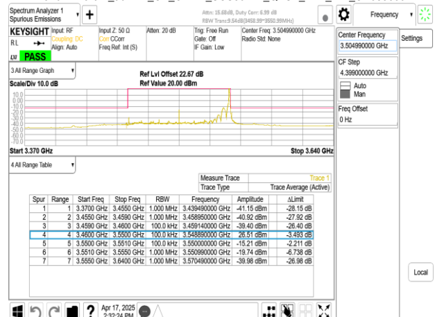
Band77-Part27_90MHz_CP_OFDM_SCS30kHz_QPSK_RB1_244_CH633666
