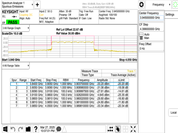
Band77-Part27_70MHz_CP_OFDM_SCS30kHz_QPSK_RB1_0_CH663000
