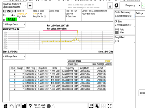
Band77-Part27_90MHz_DFT_s_OFDM_SCS30kHz_BPSK_RB1_244_CH633666
