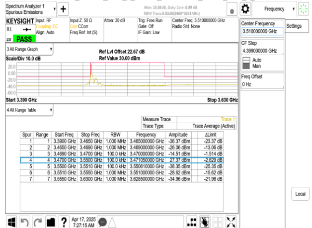
Band77-Part27_80MHz_DFT_s_OFDM_SCS30kHz_BPSK_RB1_216_CH634000
