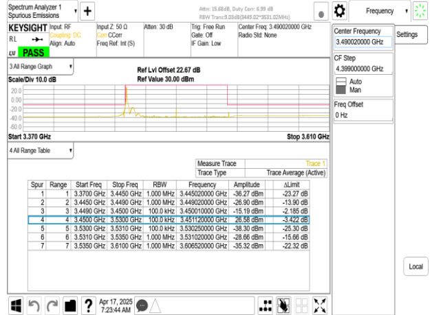
Band77-Part27_80MHz_DFT_s_OFDM_SCS30kHz_BPSK_RB1_216_CH632668
