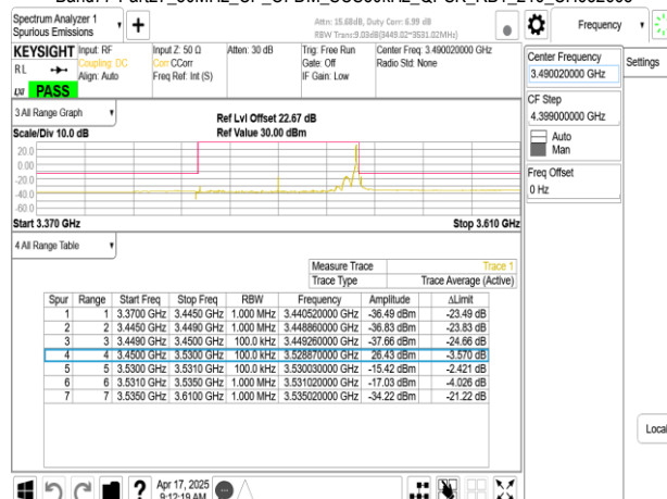
Band77-Part27_80MHz_CP_OFDM_SCS30kHz_QPSK_RB1_216_CH632668
