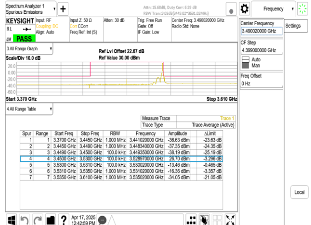
Band77-Part27_80MHz_DFT_s_OFDM_SCS30kHz_BPSK_RB1_216_CH632668
