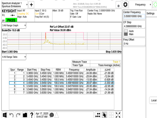
Band77-Part27_90MHz_CP_OFDM_SCS30kHz_QPSK_RB1_244_CH633334
