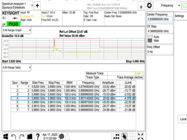
Band77-Part27_80MHz_CP_OFDM_SCS30kHz_QPSK_RB1_216_CH662666
