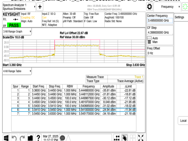
Band77-Part27_90MHz_DFT_s_OFDM_SCS30kHz_BPSK_RB1_0_CH633334
