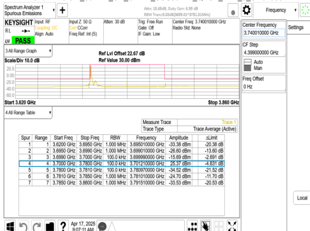
Band77-Part27_80MHz_CP_OFDM_SCS30kHz_QPSK_RB1_216_CH649334
