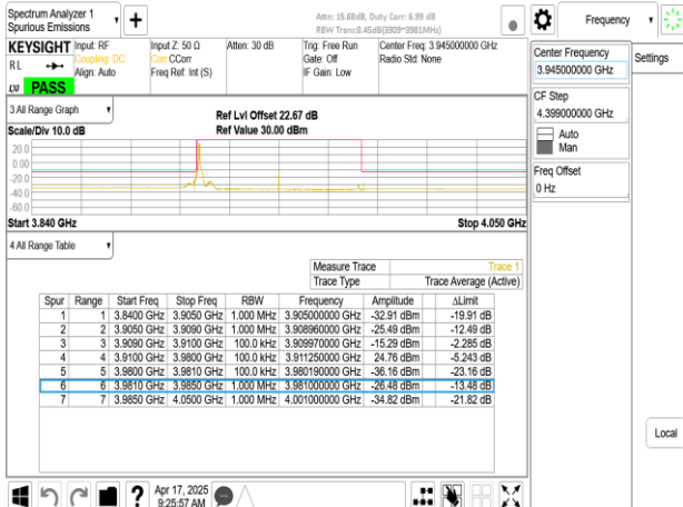
Band77-Part27_70MHz_CP_OFDM_SCS30kHz_QPSK_RB1_0_CH663000
