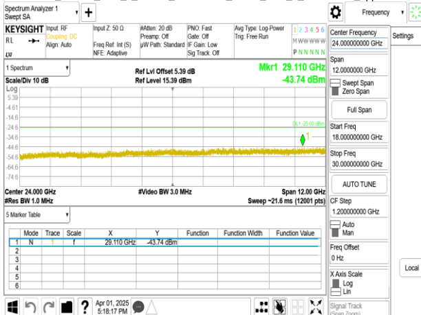
Band77-Part27_100MHz_DFT_s_OFDM_SCS30kHz_BPSK_RB1_1_CH633334_upper 18G
