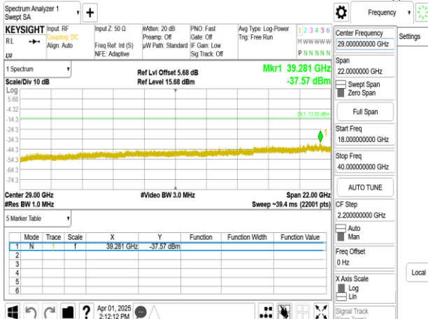
Band77-Part27_100MHz_DFT_s_OFDM_SCS30kHz_BPSK_RB1_1_CH633334_upper 18G
