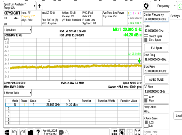
Band41_90MHz_DFT_s_OFDM_SCS30kHz_BPSK_RB1_1_CH509004_upper 18G
