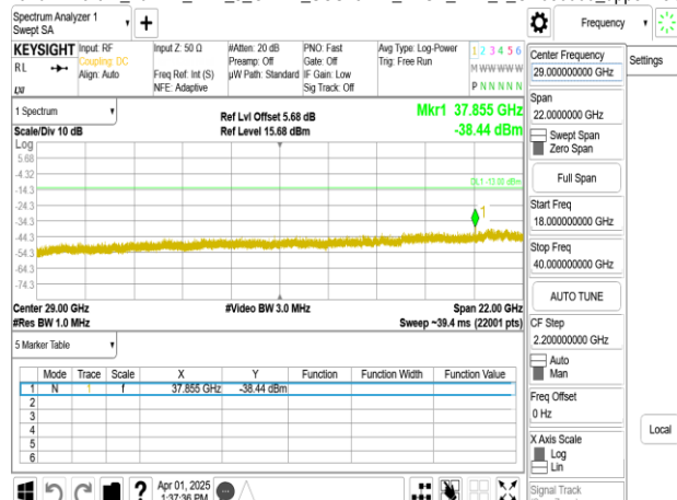
Band77-Part27_20MHz_DFT_s_OFDM_SCS15kHz_BPSK_RB1_1_CH636000_upper 18G
