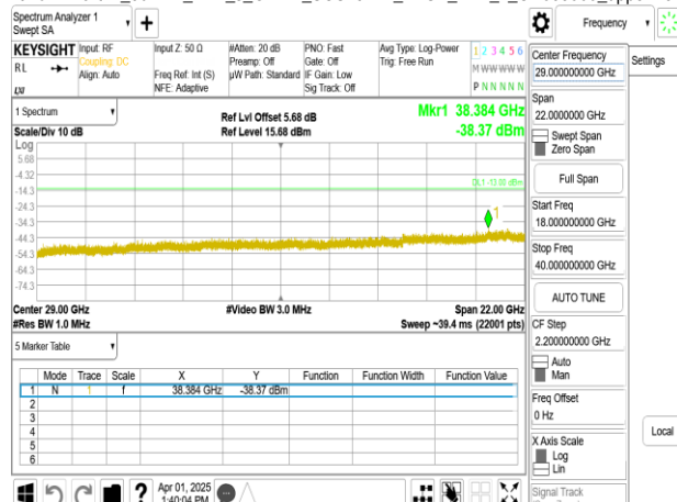
Band77-Part27_30MHz_DFT_s_OFDM_SCS15kHz_BPSK_RB1_1_CH635666_upper 18G
