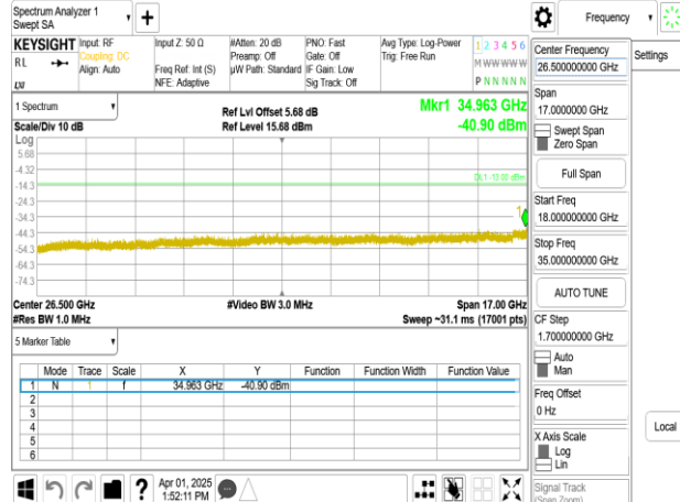
Band77-Part27_20MHz_DFT_s_OFDM_SCS30kHz_BPSK_RB1_1_CH633334_upper 18G
