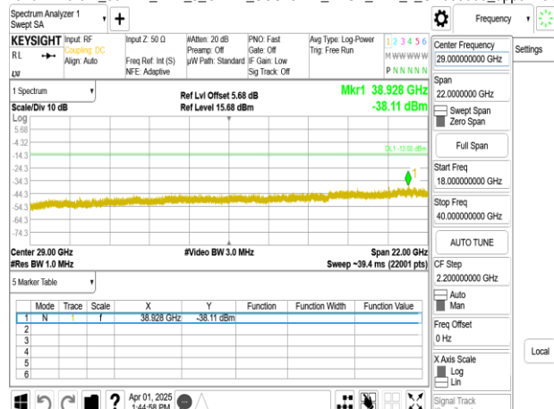
Band77-Part27_50MHz_DFT_s_OFDM_SCS15kHz_BPSK_RB1_1_CH635000_upper 18G
