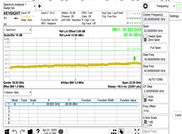
Band77-Part27_30MHz_DFT_s_OFDM_SCS30kHz_BPSK_RB1_1_CH635666_upper 18G
