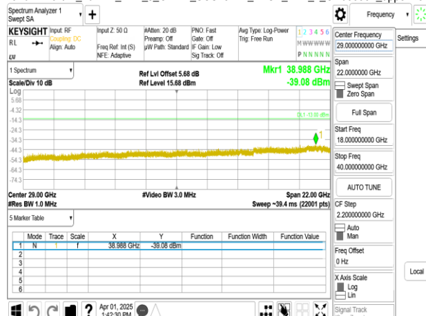
Band77-Part27_40MHz_DFT_s_OFDM_SCS15kHz_BPSK_RB1_1_CH635332_upper 18G
