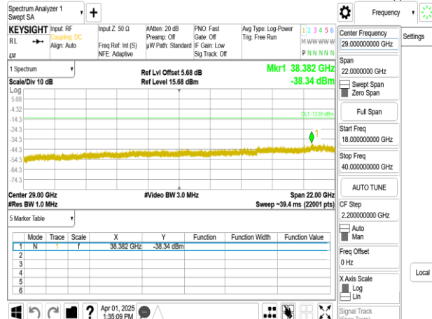
Band77-Part27_15MHz_DFT_s_OFDM_SCS15kHz_BPSK_RB1_1_CH636166_upper 18G
