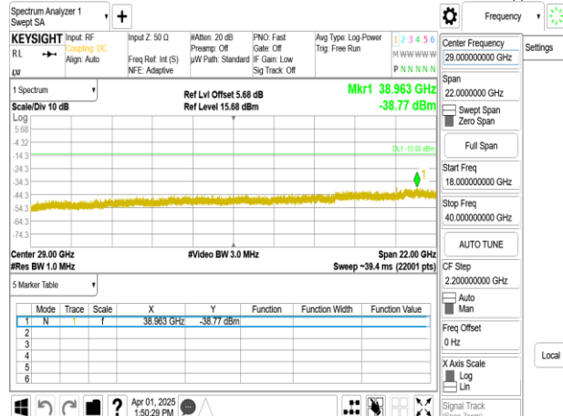
Band77-Part27_15MHz_DFT_s_OFDM_SCS30kHz_BPSK_RB1_1_CH636166_upper 18G
