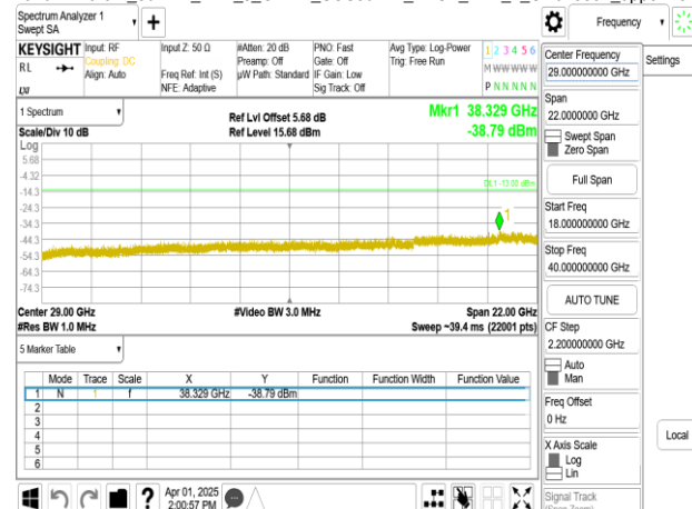
Band77-Part27_50MHz_DFT_s_OFDM_SCS30kHz_BPSK_RB1_1_CH656000_upper 18G
