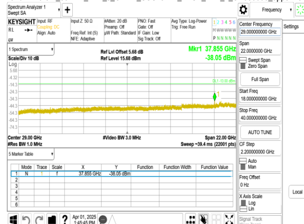
Band77-Part27_50MHz_DFT_s_OFDM_SCS15kHz_BPSK_RB1_1_CH663666_upper 18G
