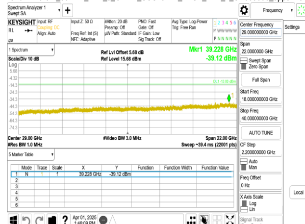
Band77-Part27_50MHz_DFT_s_OFDM_SCS15kHz_BPSK_RB1_1_CH663666_upper 18G
