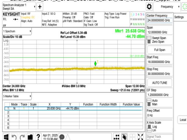
Band7_25MHz_DFT_s_OFDM_SCS15kHz_BPSK_RB1_1_CH507000_upper 18G
