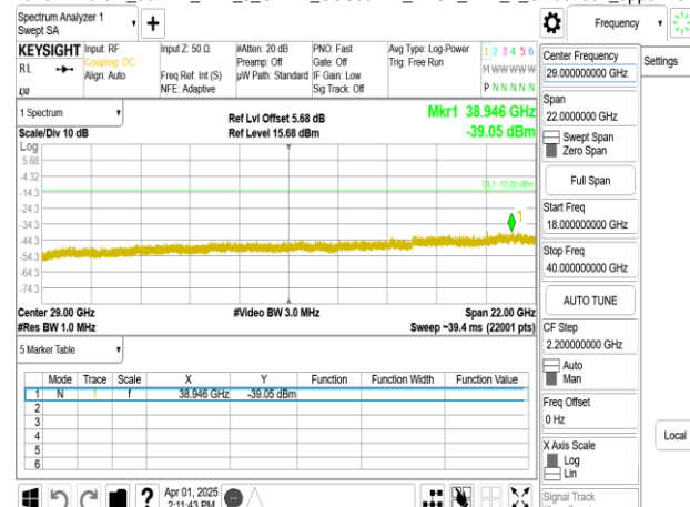
Band77-Part27_90MHz_DFT_s_OFDM_SCS30kHz_BPSK_RB1_1_CH62332_upper 18G
