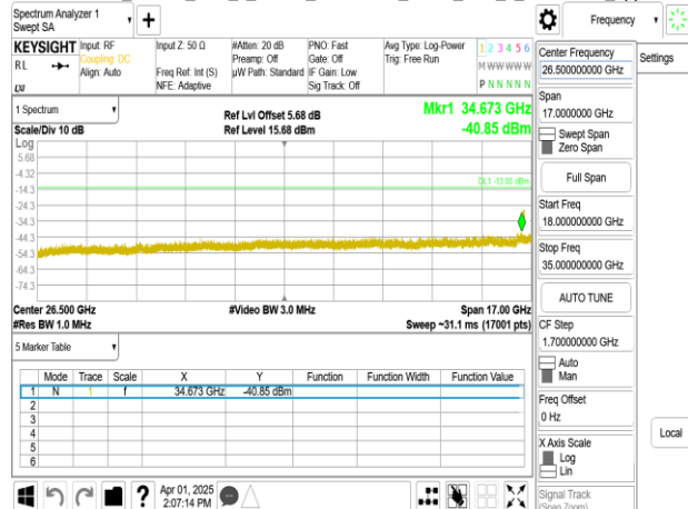
Band77-Part27_80MHz_DFT_s_OFDM_SCS30kHz_BPSK_RB1_1_CH633334_upper 18G
