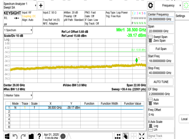
Band77-Part27_70MHz_DFT_s_OFDM_SCS30kHz_BPSK_RB1_1_CH634332_upper 18G
