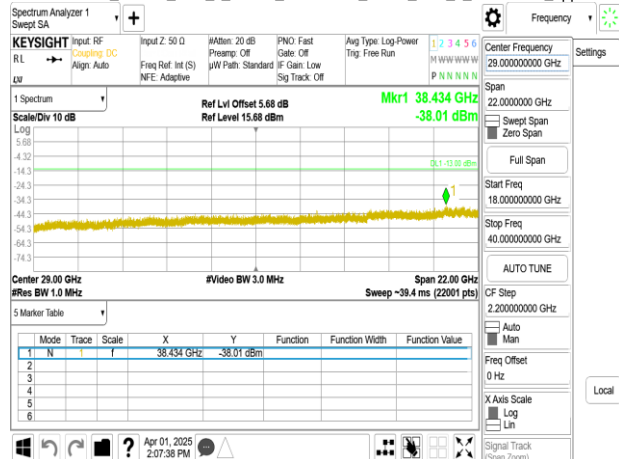
Band77-Part27_80MHz_DFT_s_OFDM_SCS30kHz_BPSK_RB1_1_CH634000_upper 18G
