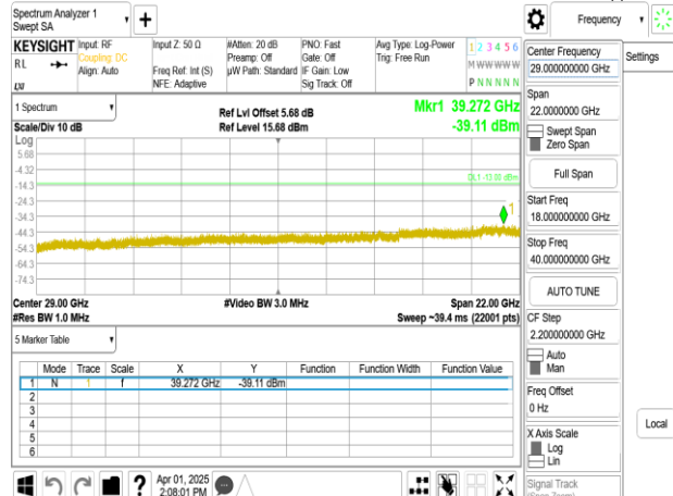
Band77-Part27_80MHz_DFT_s_OFDM_SCS30kHz_BPSK_RB1_1_CH634000_upper 18G
