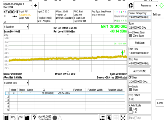
Band77-Part27_90MHz_DFT_s_OFDM_SCS30kHz_BPSK_RB1_1_CH633666_upper 18G
