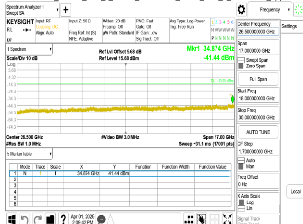
Band77-Part27_90MHz_DFT_s_OFDM_SCS30kHz_BPSK_RB1_1_CH633334_upper 18G
