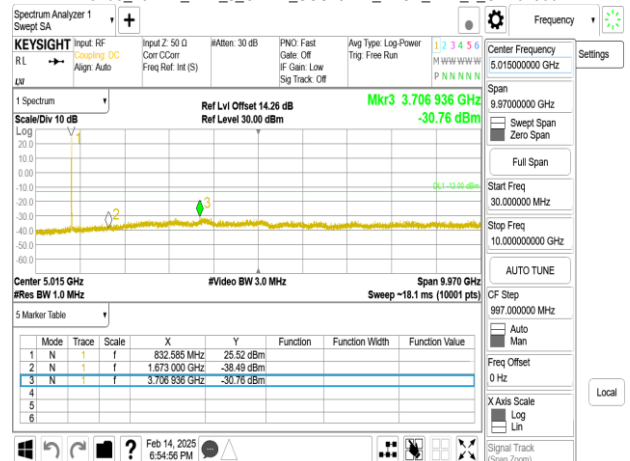
Band5_10MHz_DFT_s_OFDM_SCS15kHz_BPSK_RB1_1_CH168800
