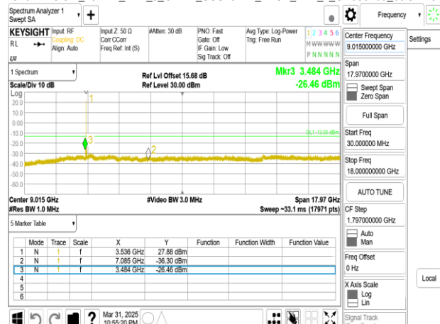
Band77-Part27_15MHz_DFT_s_OFDM_SCS15kHz_BPSK_RB1_1_CH636166_below 18G
