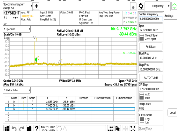
Band77-Part27_15MHz_DFT_s_OFDM_SCS30kHz_BPSK_RB1_1_CH636166_below 18G
