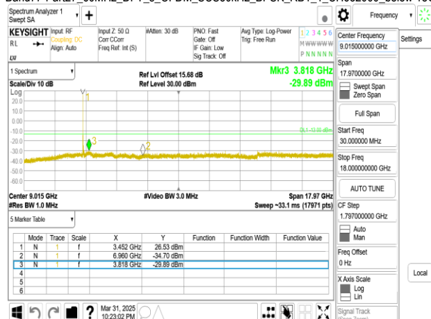
Band77-Part27_60MHz_DFT_s_OFDM_SCS30kHz_BPSK_RB1_1_CH633334_below 18G
