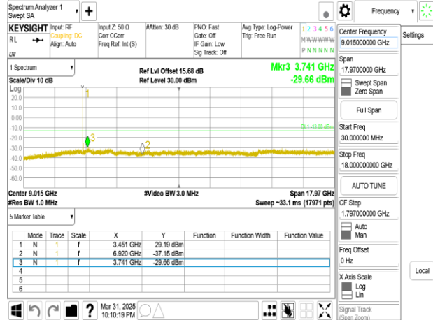
Band77-Part27_20MHz_DFT_s_OFDM_SCS30kHz_BPSK_RB1_1_CH633334_below 18G
