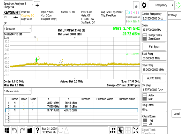
Band77-Part27_50MHz_DFT_s_OFDM_SCS15kHz_BPSK_RB1_1_CH635000_below 18G
