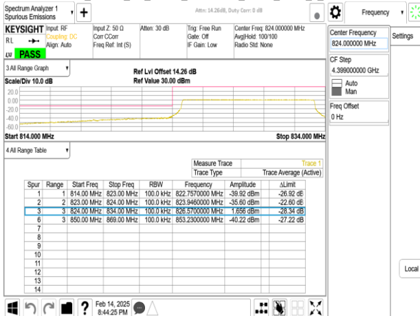
Band5_10MHz_CP_OFDM_SCS30kHz_QPSK_RB1_23_CH168800
