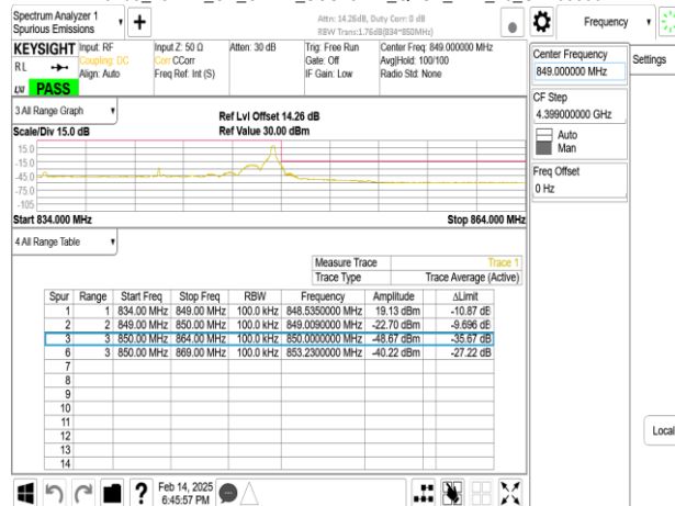
Band5_15MHz_CP_OFDM_SCS15kHz_QPSK_RB79_0_CH168300
