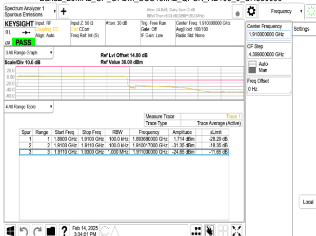
Band2_20MHz_CP_OFDM_SCS15kHz_QPSK_RB1_105_CH380000
