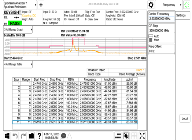
Band7_5MHz_CP_OFDM_SCS15kHz_QPSK_RB1_24_CH500500
