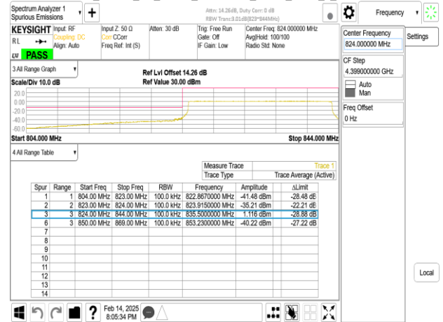
Band5_20MHz_CP_OFDM_SCS30kHz_QPSK_RB1_50_CH167800
