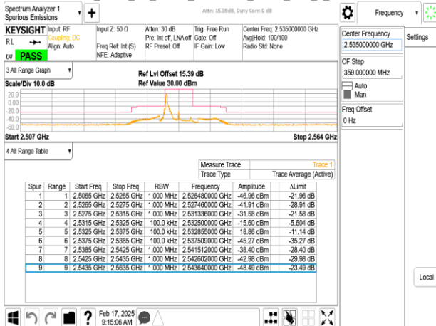
Band7_5MHz_CP_OFDM_SCS15kHz_QPSK_RB1_24_CH507000
