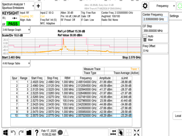
Band7_15MHz_CP_OFDM_SCS15kHz_QPSK_RB1_78_CH507000
