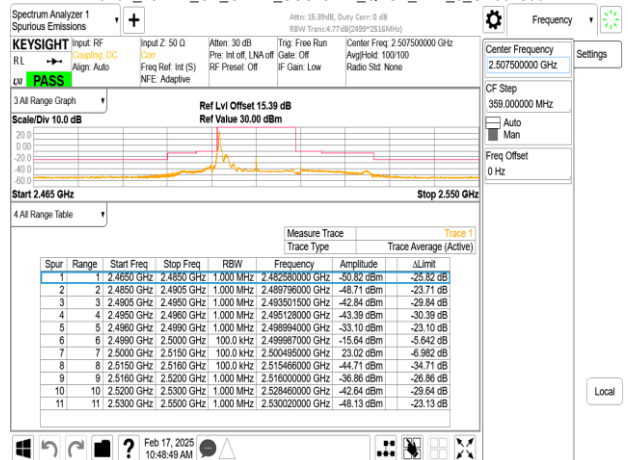
Band7_15MHz_CP_OFDM_SCS15kHz_QPSK_RB1_78_CH501500
