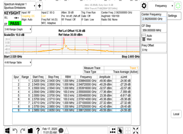
Band7_15MHz_CP_OFDM_SCS15kHz_QPSK_RB1_78_CH512500
