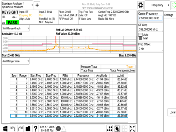
Band7_50MHz_CP_OFDM_SCS15kHz_QPSK_RB1_269_CH507000
