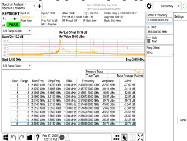
Band7_40MHz_CP_OFDM_SCS30kHz_QPSK_RB1_105_CH507000
