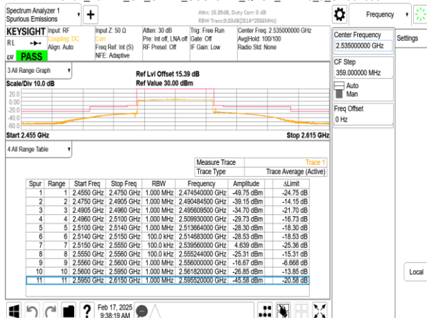
Band7_40MHz_CP_OFDM_SCS15kHz_QPSK_RB216_0_CH507000
