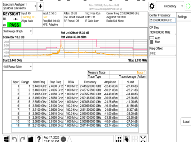
Band7_50MHz_CP_OFDM_SCS30kHz_QPSK_RB1_132_CH507000
