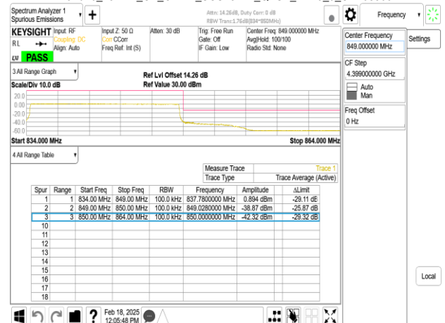
Band26_15MHz_CP_OFDM_SCS15kHz_QPSK_RB79_0_CH168300
