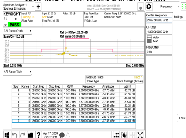
Band38_15MHz_CP_OFDM_SCS15kHz_QPSK_RB1_78_CH515500
