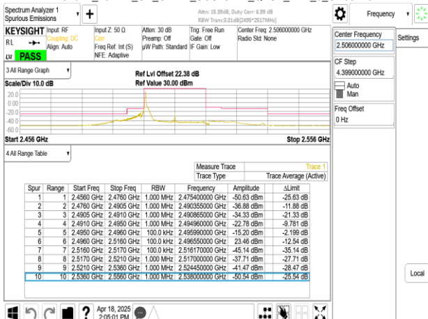
Band41_20MHz_CP_OFDM_SCS15kHz_QPSK_RB1_105_CH501204
