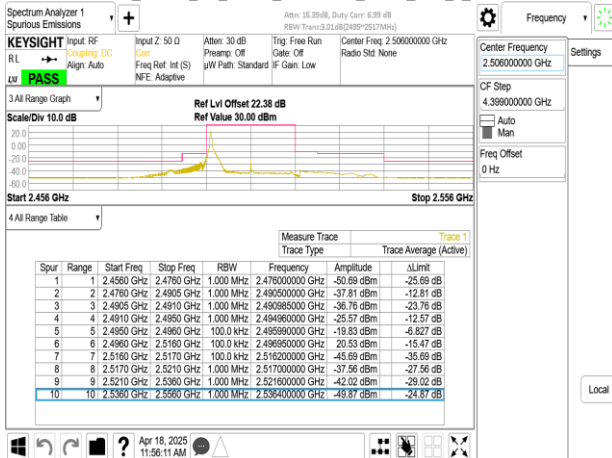
Band41_20MHz_CP_OFDM_SCS30kHz_QPSK_RB1_50_CH501204
