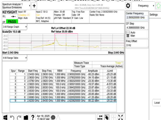
Band41_20MHz_CP_OFDM_SCS30kHz_QPSK_RB1_50_CH518604
