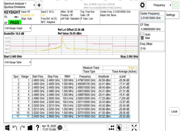
Band41_20MHz_CP_OFDM_SCS30kHz_QPSK_RB1_50_CH502002
