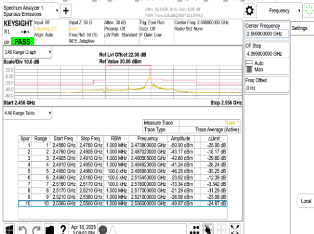
Band41_20MHz_CP_OFDM_SCS15kHz_QPSK_RB1_105_CH501204
