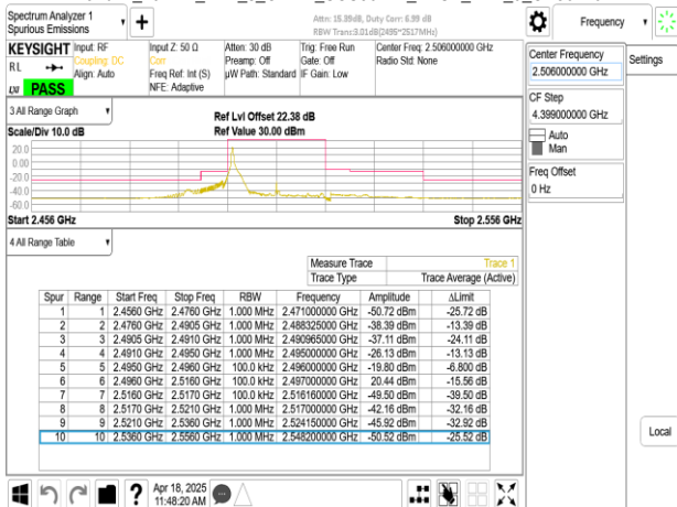
Band41_20MHz_DFT_s_OFDM_SCS30kHz_BPSK_RB1_50_CH501204
