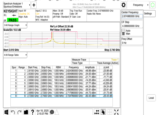
Band41_30MHz_CP_OFDM_SCS15kHz_QPSK_RB1_159_CH534996
