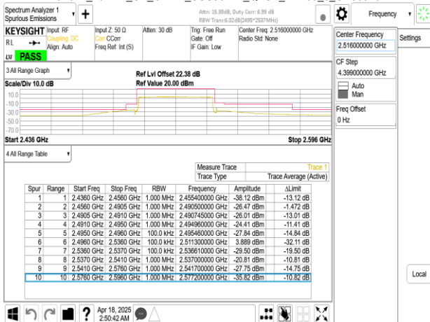
Band41_40MHz_CP_OFDM_SCS30kHz_QPSK_RB1_0_CH503202
