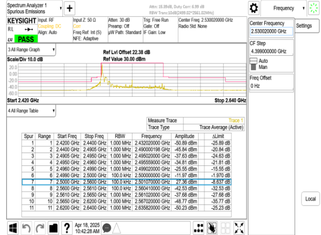
Band41_60MHz_DFT_s_OFDM_SCS30kHz_BPSK_RB1_161_CH506004
