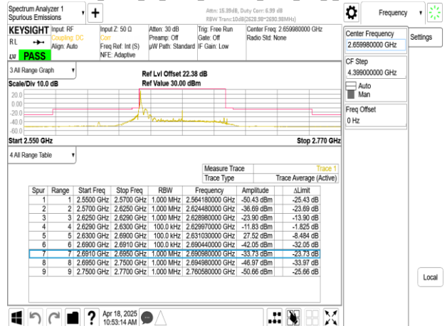
Band41_60MHz_CP_OFDM_SCS30kHz_QPSK_RB1_161_CH51996
