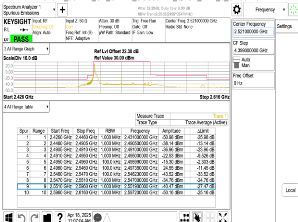
Band41_50MHz_CP_OFDM_SCS30kHz_QPSK_RB1_132_CH504204
