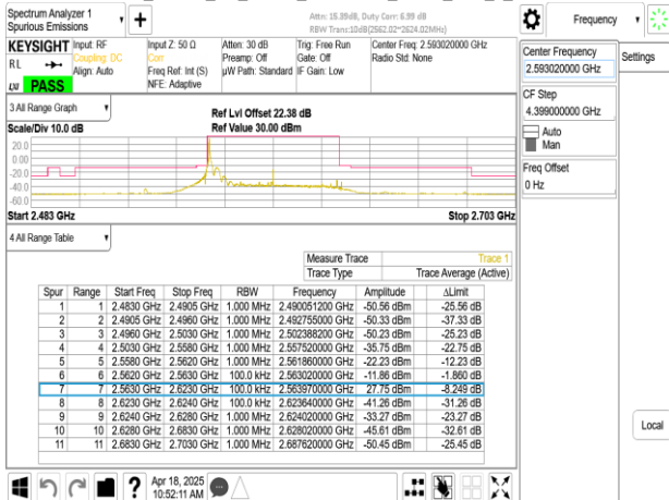
Band41_60MHz_CP_OFDM_SCS30kHz_QPSK_RB1_161_CH518604
