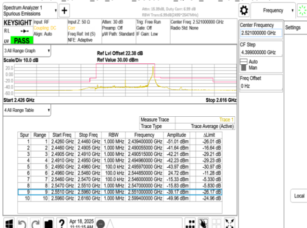
Band41_50MHz_CP_OFDM_SCS30kHz_QPSK_RB1_132_CH504204
