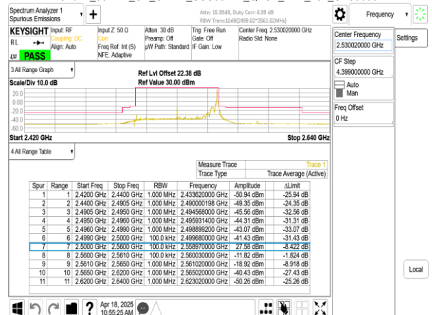
Band41_60MHz_CP_OFDM_SCS30kHz_QPSK_RB1_161_CH506004
