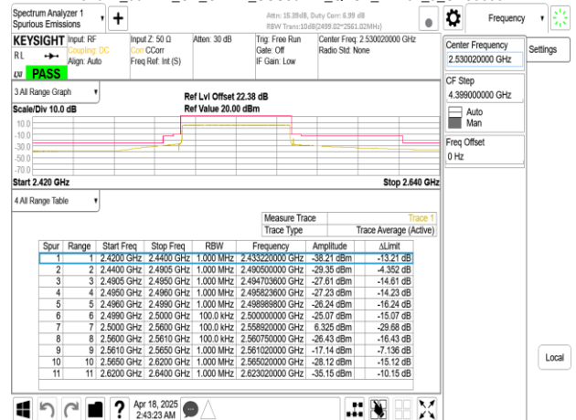
Band41_60MHz_CP_OFDM_SCS30kHz_QPSK_RB1_0_CH506004
