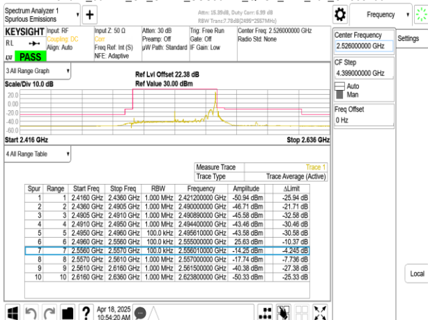
Band41_60MHz_CP_OFDM_SCS30kHz_QPSK_RB1_161_CH505200
