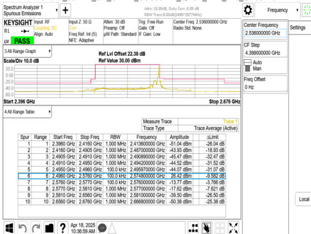
Band41_80MHz_CP_OFDM_SCS30kHz_QPSK_RB217_0_CH507204
