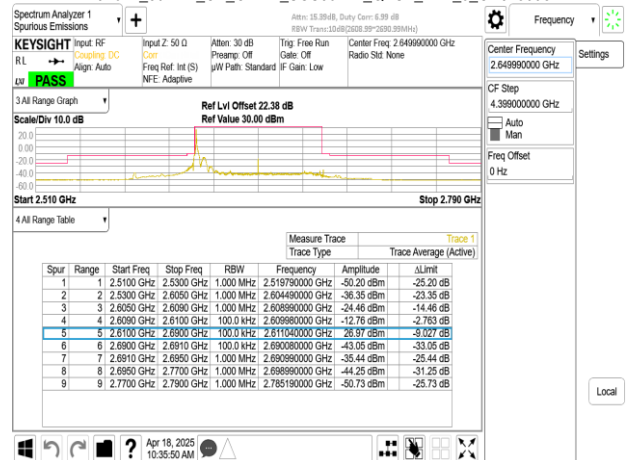
Band41_80MHz_CP_OFDM_SCS30kHz_QPSK_RB1_216_CH529998
