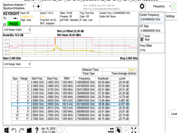
Band41_90MHz_CP_OFDM_SCS30kHz_QPSK_RB1_244_CH528996
