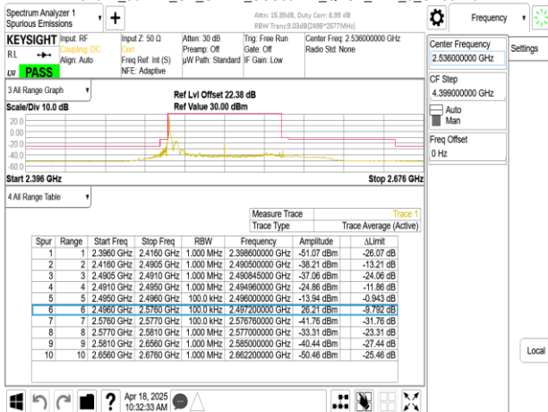
Band41_80MHz_CP_OFDM_SCS30kHz_QPSK_RB1_216_CH507204
