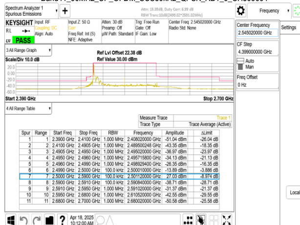
Band41_90MHz_CP_OFDM_SCS30kHz_QPSK_RB1_244_CH509004
