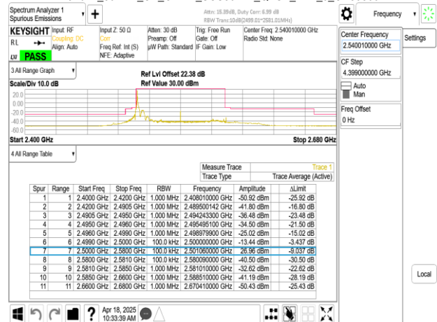
Band41_80MHz_CP_OFDM_SCS30kHz_QPSK_RB1_216_CH508002
