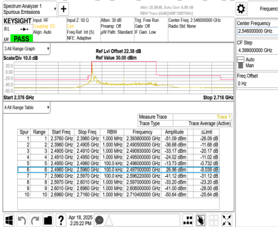
Band41_100MHz_CP_OFDM_SCS30kHz_QPSK_RB1_272_CH509202
