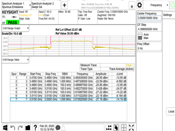
Band77-Part27_20MHz_CP_OFDM_SCS15kHz_QPSK_RB1_0_CH633334
