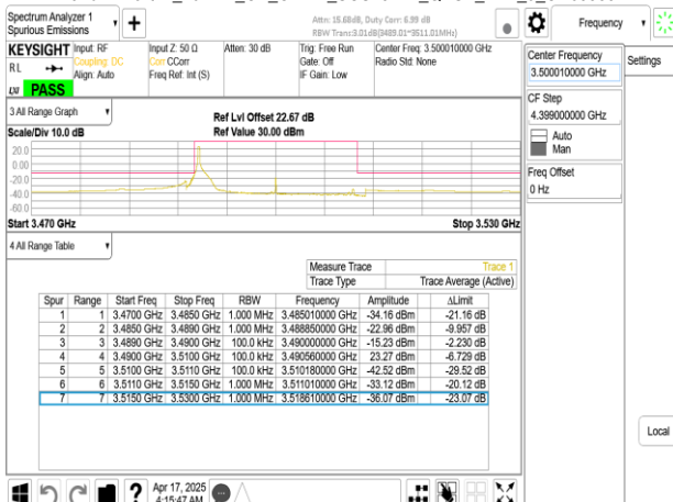
Band77-Part27_20MHz_CP_OFDM_SCS15kHz_QPSK_RB1_0_CH633334
