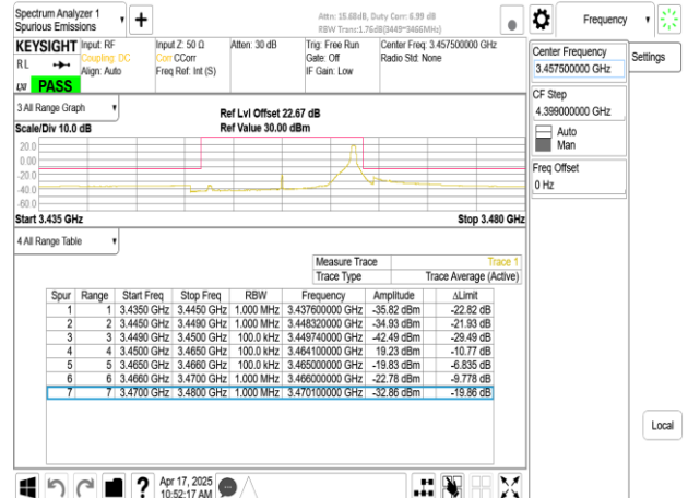
Band77-Part27_15MHz_CP_OFDM_SCS30kHz_QPSK_RB1_37_CH630500
