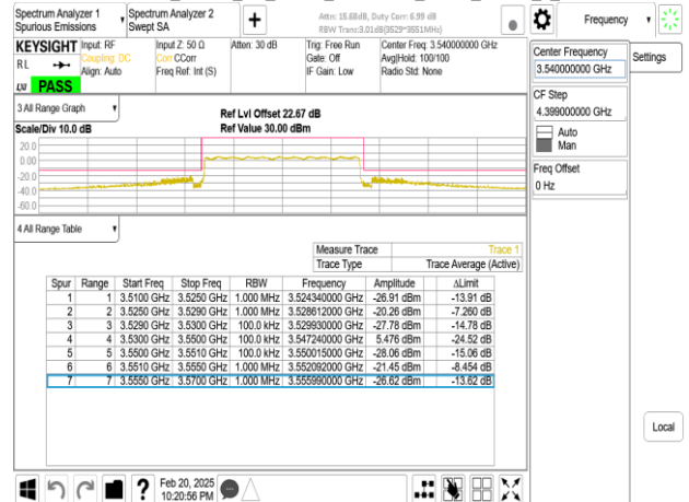
Band77-Part27_20MHz_CP_OFDM_SCS15kHz_QPSK_RB1_0_CH636000
