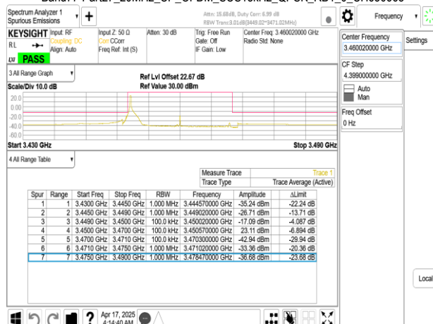
Band77-Part27_20MHz_CP_OFDM_SCS15kHz_QPSK_RB1_0_CH630668
