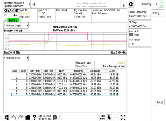
Band77-Part27_15MHz_CP_OFDM_SCS30kHz_QPSK_RB1_37_CH630500
