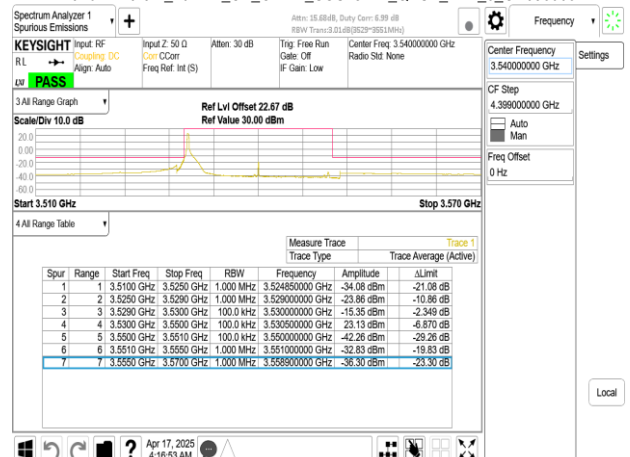
Band77-Part27_20MHz_CP_OFDM_SCS15kHz_QPSK_RB1_0_CH636000
