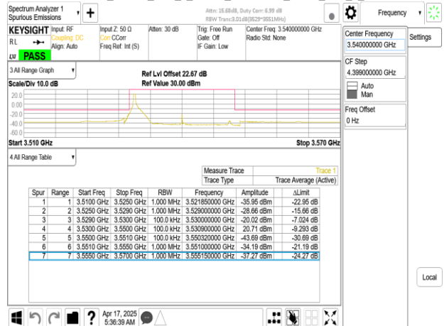
Band77-Part27_20MHz_DFT_s_OFDM_SCS30kHz_BPSK_RB1_50_CH636000
