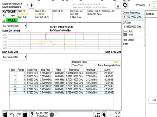
Band77-Part27_20MHz_DFT_s_OFDM_SCS30kHz_BPSK_RB1_50_CH647334
