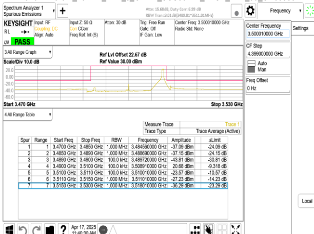
Band77-Part27_20MHz_DFT_s_OFDM_SCS30kHz_BPSK_RB1_50_CH633334
