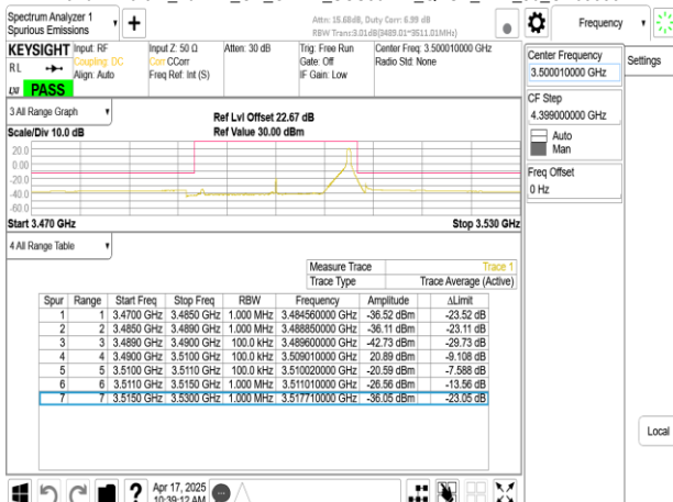
Band77-Part27_20MHz_CP_OFDM_SCS30kHz_QPSK_RB1_50_CH633334
