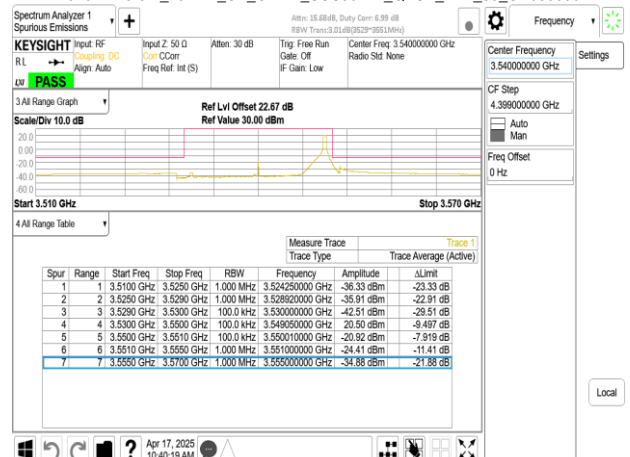
Band77-Part27_20MHz_CP_OFDM_SCS30kHz_QPSK_RB1_50_CH636000
