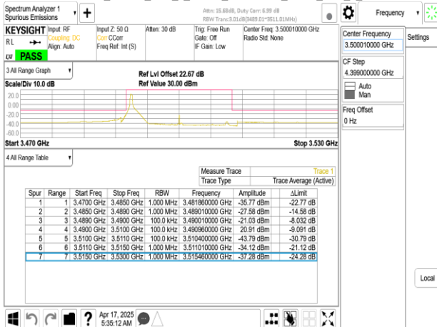
Band77-Part27_20MHz_DFT_s_OFDM_SCS30kHz_BPSK_RB1_50_CH633334
