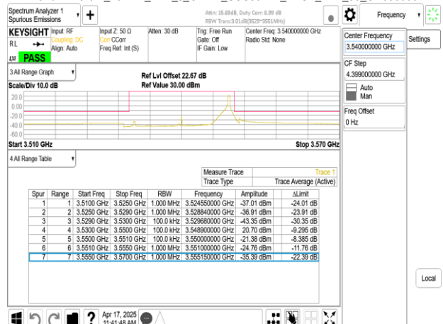
Band77-Part27_20MHz_DFT_s_OFDM_SCS30kHz_BPSK_RB1_50_CH636000
