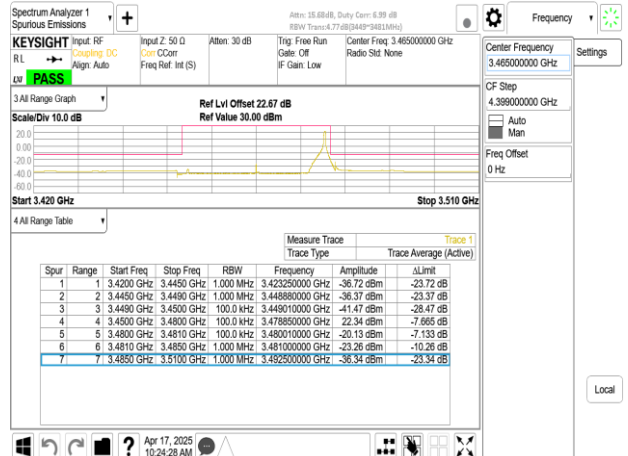
Band77-Part27_30MHz_CP_OFDM_SCS30kHz_QPSK_RB1_77_CH631000
