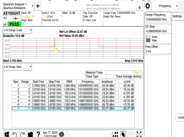
Band77-Part27_50MHz_CP_OFDM_SCS15kHz_QPSK_RB1_269_CH656000
