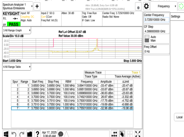
Band77-Part27_50MHz_CP_OFDM_SCS15kHz_QPSK_RB1_269_CH648334
