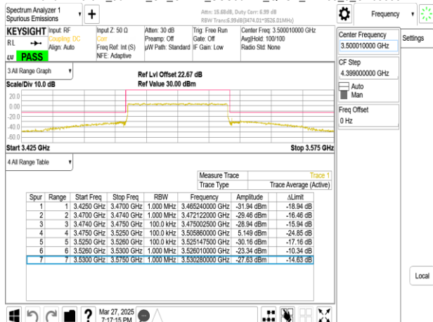
Band77-Part27_50MHz_CP_OFDM_SCS30kHz_QPSK_RB1_0_CH633334
