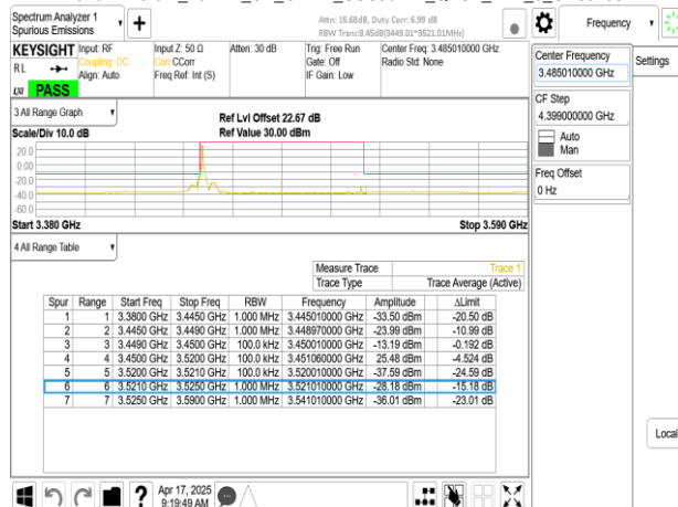
Band77-Part27_70MHz_CP_OFDM_SCS30kHz_QPSK_RB1_0_CH632334
