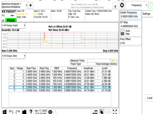
Band77-Part27_70MHz_CP_OFDM_SCS30kHz_QPSK_RB1_0_CH633334
