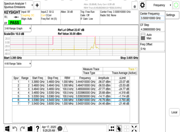
Band77-Part27_70MHz_CP_OFDM_SCS30kHz_QPSK_RB189_0_CH634332
