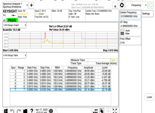
Band77-Part27_60MHz_CP_OFDM_SCS30kHz_QPSK_RB1_0_CH634666
