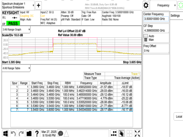
Band77-Part27_70MHz_CP_OFDM_SCS30kHz_QPSK_RB1_0_CH633334
