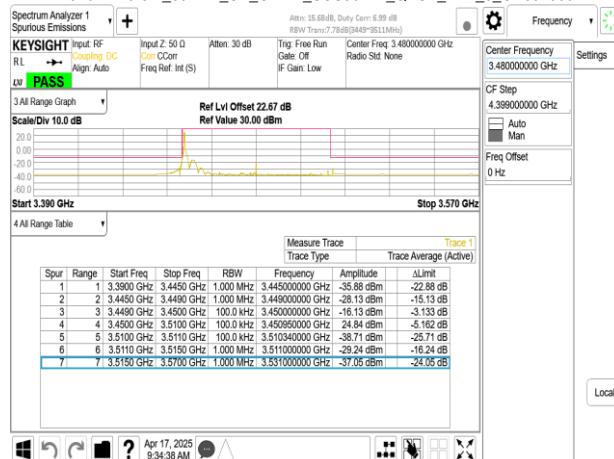
Band77-Part27_60MHz_CP_OFDM_SCS30kHz_QPSK_RB1_0_CH632000
