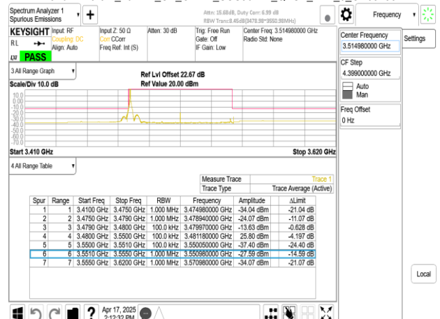
Band77-Part27_70MHz_CP_OFDM_SCS30kHz_QPSK_RB1_0_CH634332
