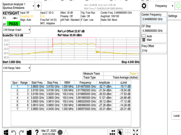
Band77-Part27_60MHz_CP_OFDM_SCS30kHz_QPSK_RB1_0_CH663332
