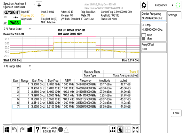
Band77-Part27_60MHz_CP_OFDM_SCS30kHz_QPSK_RB1_0_CH634666
