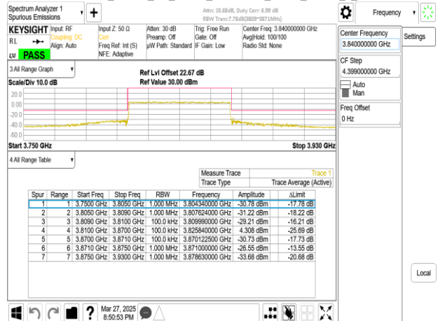
Band77-Part27_60MHz_CP_OFDM_SCS30kHz_QPSK_RB1_0_CH656000
