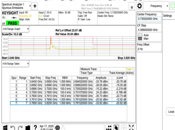
Band77-Part27_60MHz_CP_OFDM_SCS30kHz_QPSK_RB1_0_CH648668
