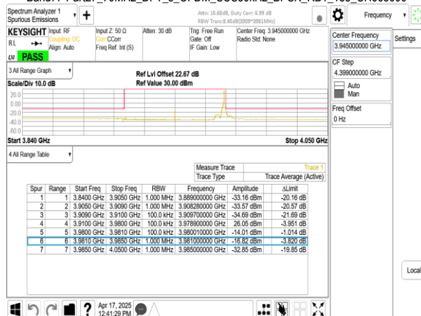
Band77-Part27_70MHz_CP_OFDM_SCS30kHz_QPSK_RB189_0_CH632334
