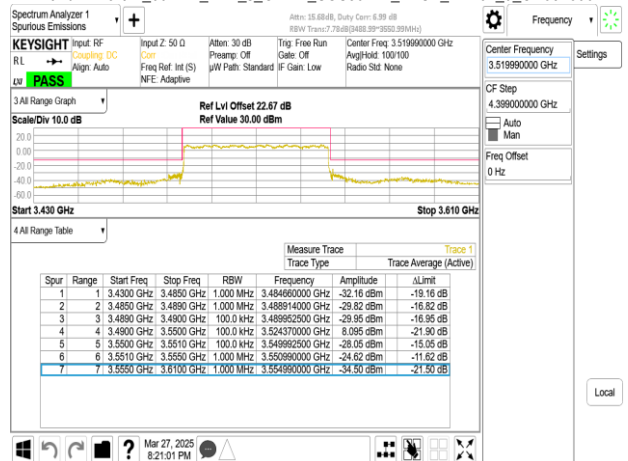
Band77-Part27_60MHz_DFT_s_OFDM_SCS30kHz_BPSK_RB1_0_CH634666
