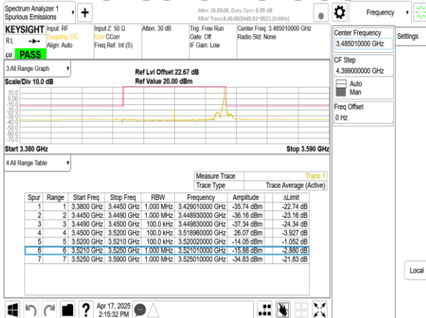
Band77-Part27_70MHz_CP_OFDM_SCS30kHz_QPSK_RB189_0_CH633334
