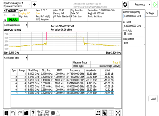
Band77-Part27_70MHz_CP_OFDM_SCS30kHz_QPSK_RB1_0_CH634332
