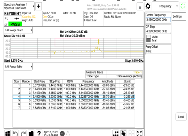
Band77-Part27_80MHz_DFT_s_OFDM_SCS30kHz_BPSK_RB1_216_CH632668
