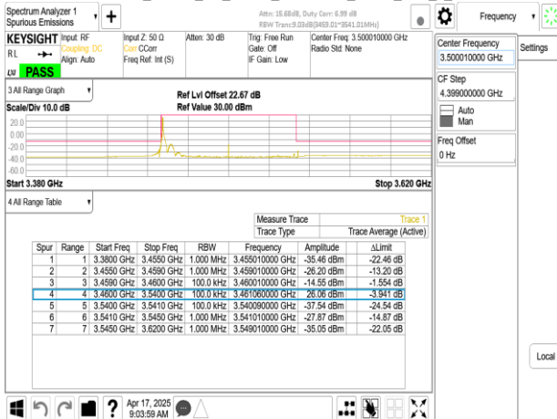
Band77-Part27_80MHz_CP_OFDM_SCS30kHz_QPSK_RB1_216_CH633334
