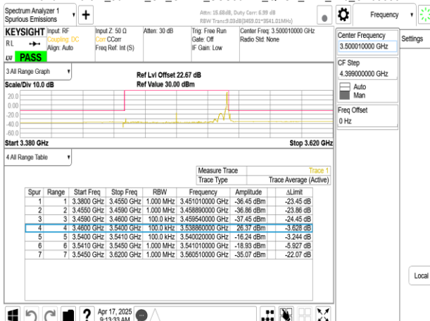
Band77-Part27_80MHz_CP_OFDM_SCS30kHz_QPSK_RB1_216_CH633334
