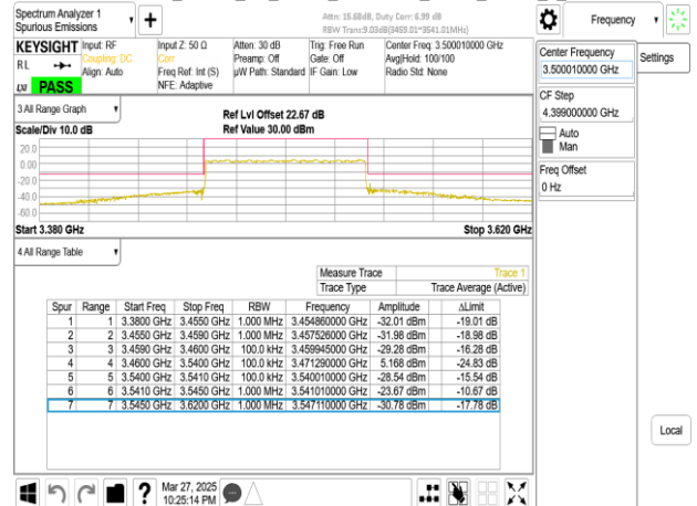
Band77-Part27_80MHz_CP_OFDM_SCS30kHz_QPSK_RB1_0_CH634000
