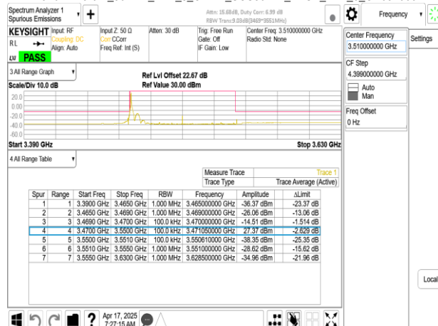
Band77-Part27_80MHz_DFT_s_OFDM_SCS30kHz_BPSK_RB1_216_CH634000
