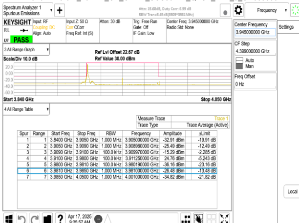
Band77-Part27_70MHz_CP_OFDM_SCS30kHz_QPSK_RB1_0_CH663000
