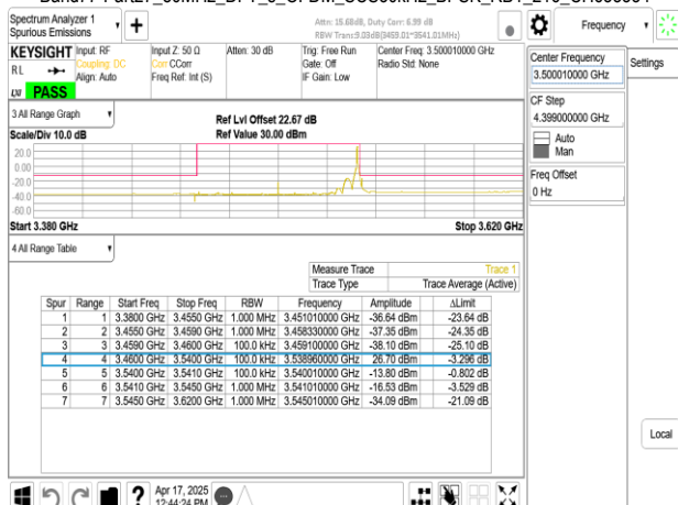
Band77-Part27_80MHz_DFT_s_OFDM_SCS30kHz_BPSK_RB1_216_CH633334
