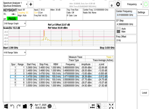
Band77-Part27_80MHz_CP_OFDM_SCS30kHz_QPSK_RB1_216_CH634000
