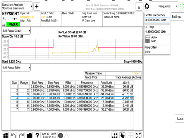
Band77-Part27_80MHz_CP_OFDM_SCS30kHz_QPSK_RB1_216_CH662666
