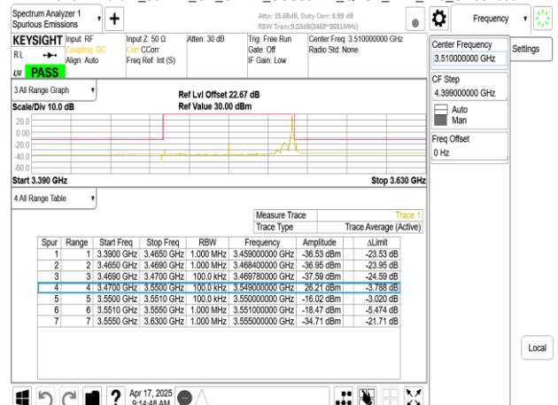
Band77-Part27_80MHz_CP_OFDM_SCS30kHz_QPSK_RB1_216_CH634000
