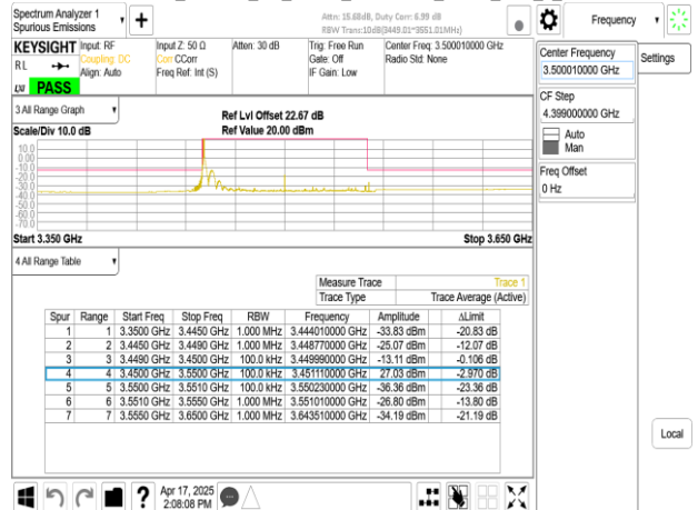
Band77-Part27_100MHz_CP_OFDM_SCS30kHz_QPSK_RB1_272_CH633334
