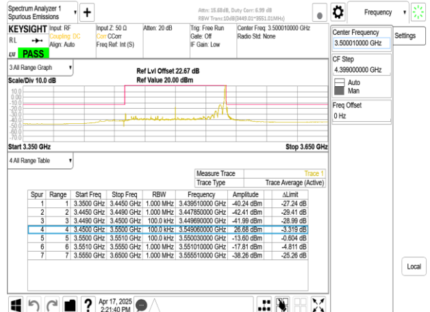
Band77-Part27_100MHz_CP_OFDM_SCS30kHz_QPSK_RB1_272_CH633334
