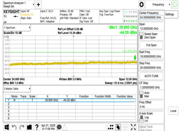
Band41_90MHz_DFT_s_OFDM_SCS30kHz_BPSK_RB1_1_CH509004_upper 18G
