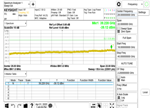
Band77-Part27_50MHz_DFT_s_OFDM_SCS15kHz_BPSK_RB1_1_CH663666_upper 18G
