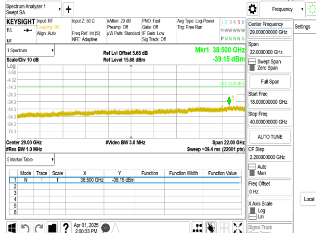
Band77-Part27_50MHz_DFT_s_OFDM_SCS30kHz_BPSK_RB1_1_CH635000_upper 18G
