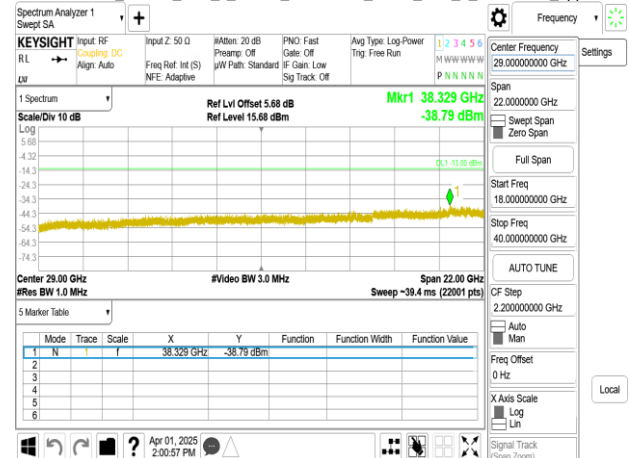
Band77-Part27_50MHz_DFT_s_OFDM_SCS30kHz_BPSK_RB1_1_CH656000_upper 18G
