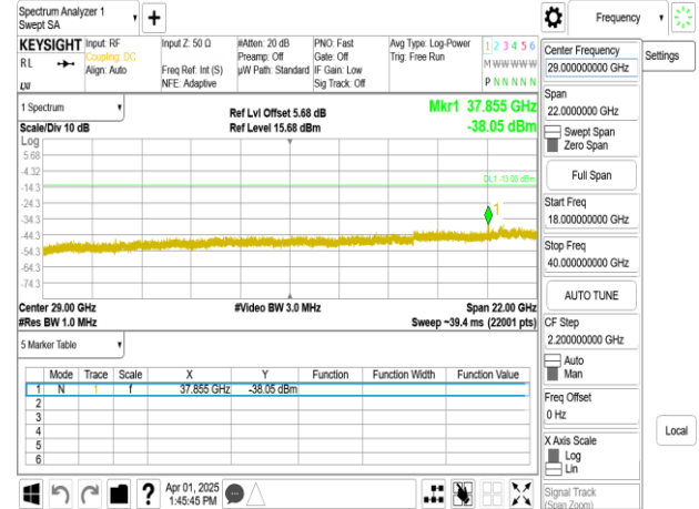
Band77-Part27_50MHz_DFT_s_OFDM_SCS15kHz_BPSK_RB1_1_CH663666_upper 18G
