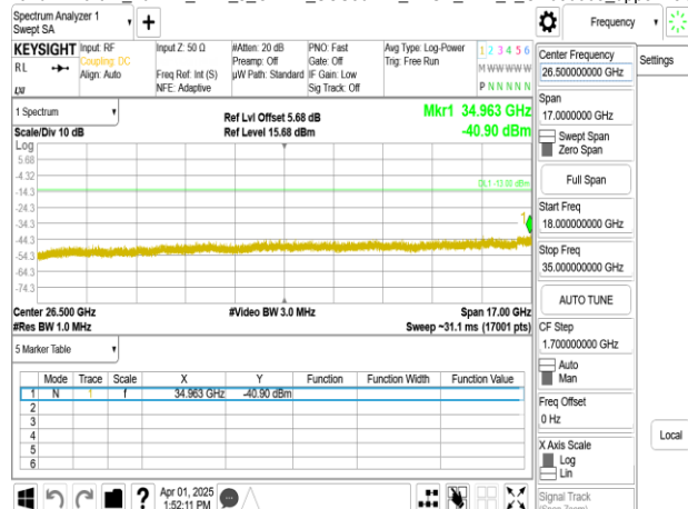
Band77-Part27_20MHz_DFT_s_OFDM_SCS30kHz_BPSK_RB1_1_CH633334_upper 18G
