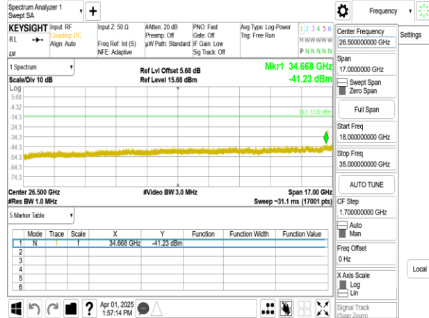
Band77-Part27_40MHz_DFT_s_OFDM_SCS30kHz_BPSK_RB1_1_CH633334_upper 18G
