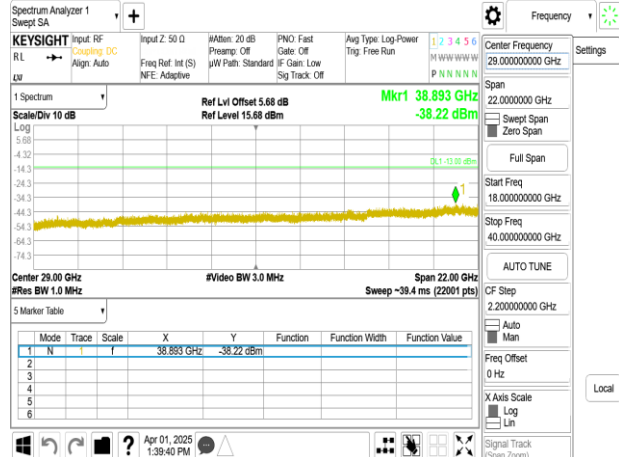
Band77-Part27_30MHz_DFT_s_OFDM_SCS15kHz_BPSK_RB1_1_CH635666_upper 18G
