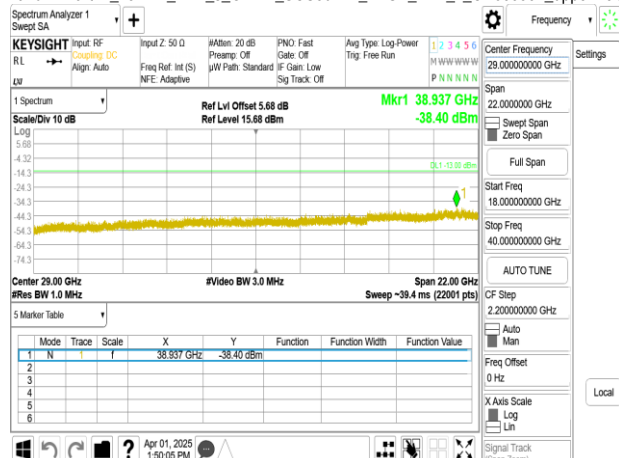
Band77-Part27_15MHz_DFT_s_OFDM_SCS30kHz_BPSK_RB1_1_CH636166_upper 18G
