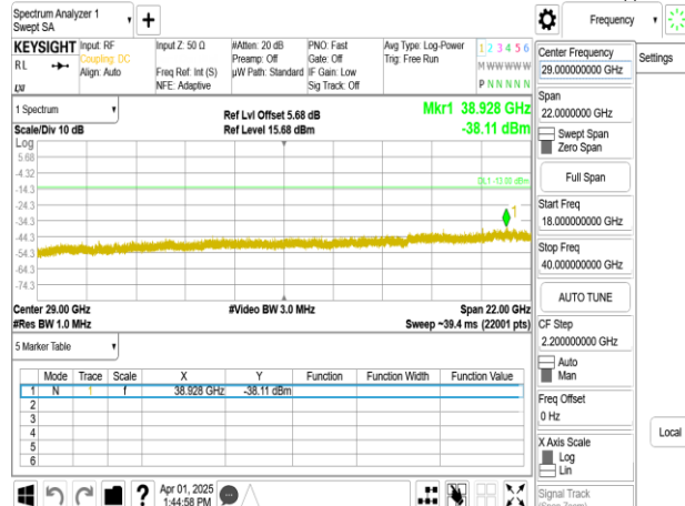
Band77-Part27_50MHz_DFT_s_OFDM_SCS15kHz_BPSK_RB1_1_CH635000_upper 18G
