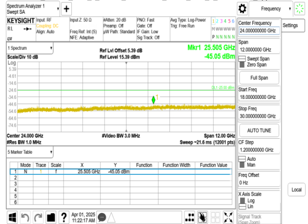
Band7_20MHz_DFT_s_OFDM_SCS30kHz_BPSK_RB1_1_CH507000_upper 18G
