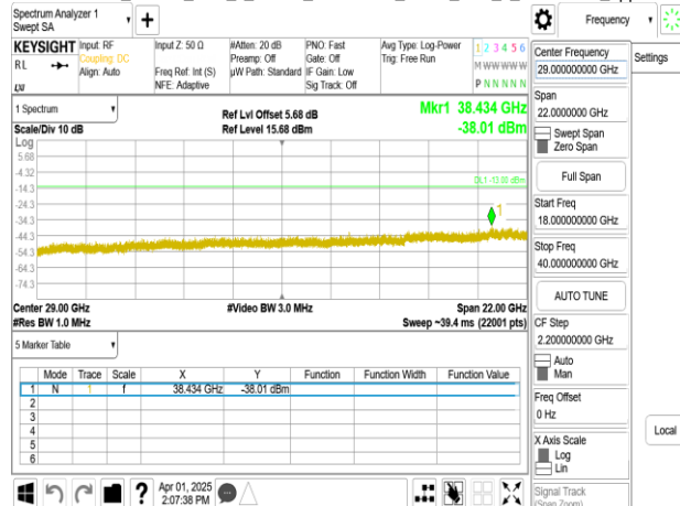
Band77-Part27_80MHz_DFT_s_OFDM_SCS30kHz_BPSK_RB1_1_CH634000_upper 18G
