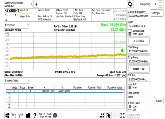
Band77-Part27_60MHz_DFT_s_OFDM_SCS30kHz_BPSK_RB1_1_CH656000_upper 18G
