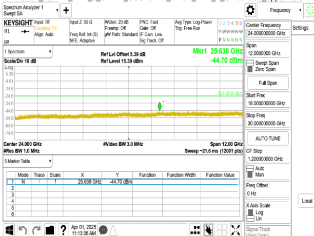
Band7_25MHz_DFT_s_OFDM_SCS15kHz_BPSK_RB1_1_CH507000_upper 18G
