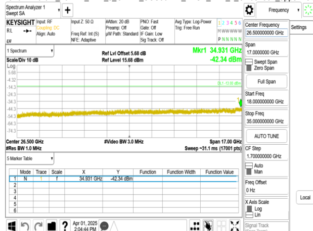
Band77-Part27_70MHz_DFT_s_OFDM_SCS30kHz_BPSK_RB1_1_CH633334_upper 18G
