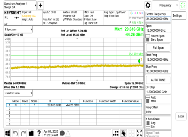
Band7_20MHz_DFT_s_OFDM_SCS30kHz_BPSK_RB1_1_CH512000_upper 18G
