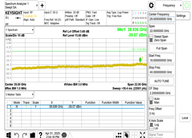
Band77-Part27_60MHz_DFT_s_OFDM_SCS30kHz_BPSK_RB1_1_CH633332_upper 18G
