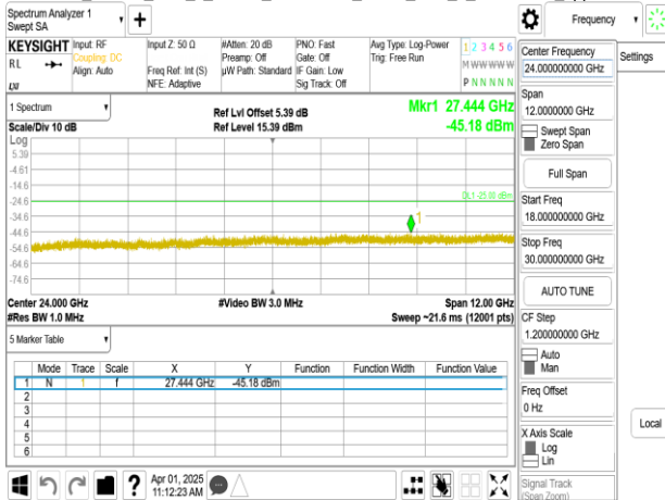
Band7_20MHz_DFT_s_OFDM_SCS15kHz_BPSK_RB1_1_CH507000_upper 18G
