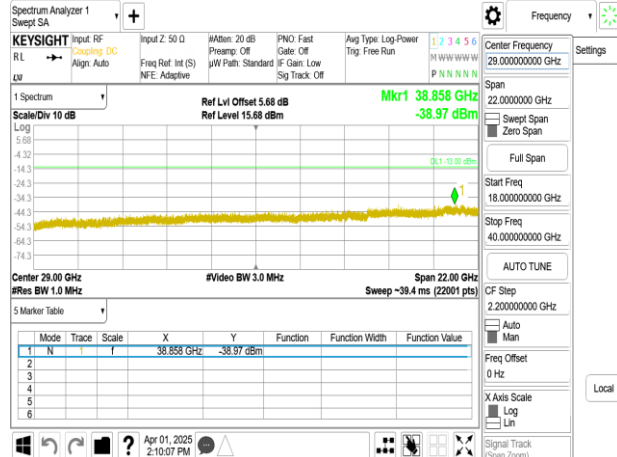
Band77-Part27_90MHz_DFT_s_OFDM_SCS30kHz_BPSK_RB1_1_CH633666_upper 18G
