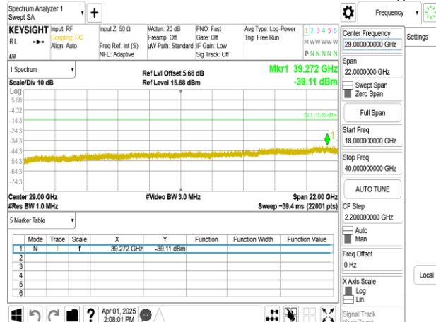
Band77-Part27_80MHz_DFT_s_OFDM_SCS30kHz_BPSK_RB1_1_CH634000_upper 18G
