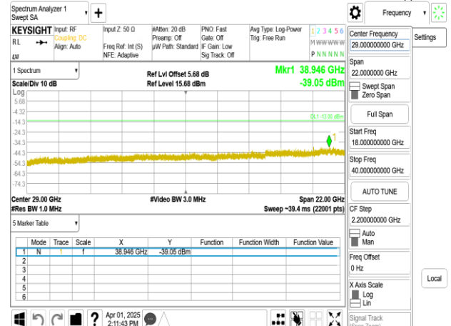
Band77-Part27_90MHz_DFT_s_OFDM_SCS30kHz_BPSK_RB1_1_CH62332_upper 18G
