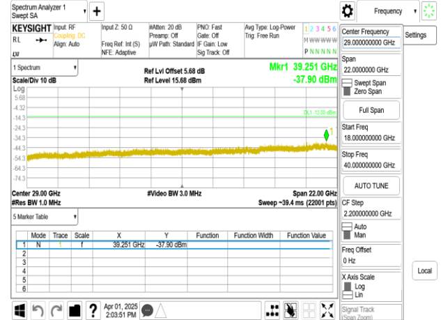
Band77-Part27_60MHz_DFT_s_OFDM_SCS30kHz_BPSK_RB1_1_CH633332_upper 18G
