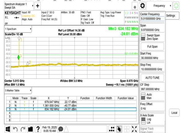
Band71_10MHz_DFT_s_OFDM_SCS30kHz_BPSK_RB1_1.CH136600
