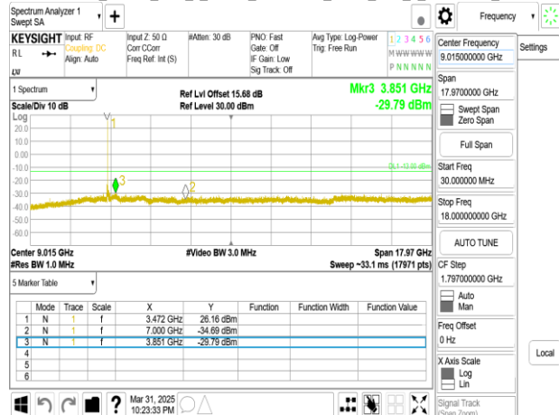
Band77-Part27_60MHz_DFT_s_OFDM_SCS30kHz_BPSK_RB1_1_CH634666_below 18G
