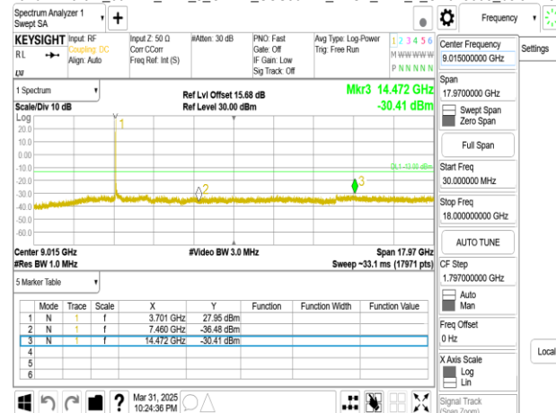
Band77-Part27_60MHz_DFT_s_OFDM_SCS30kHz_BPSK_RB1_1_CH656000_below 18G
