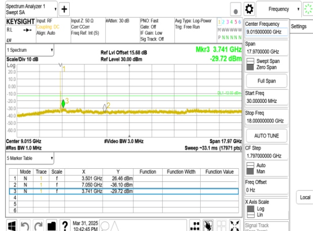
Band77-Part27_50MHz_DFT_s_OFDM_SCS15kHz_BPSK_RB1_1_CH635000_below 18G
