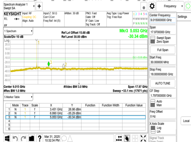
Band77-Part27_90MHz_DFT_s_OFDM_SCS30kHz_BPSK_RB1_1_CH633334_below 18G
