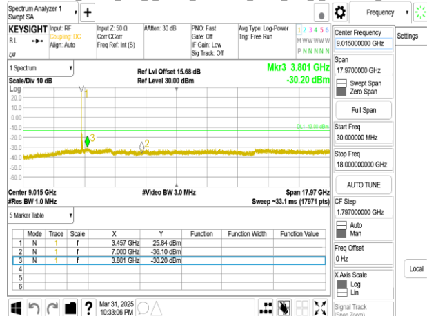
Band77-Part27_90MHz_DFT_s_OFDM_SCS30kHz_BPSK_RB1_1_CH633666_below 18G
