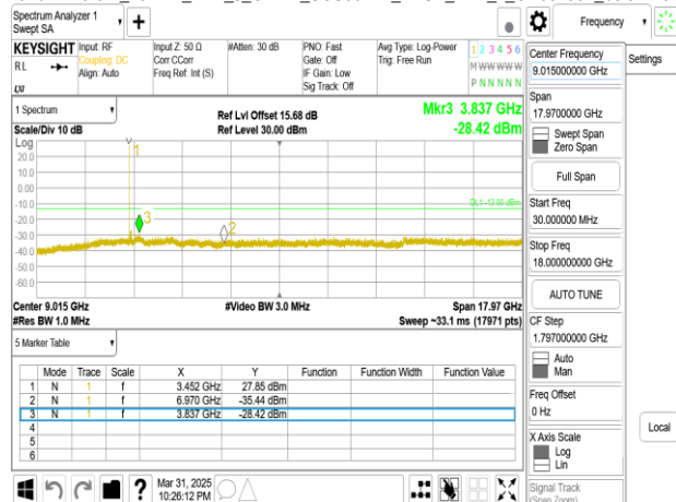
Band77-Part27_70MHz_DFT_s_OFDM_SCS30kHz_BPSK_RB1_1_CH633334_below 18G
