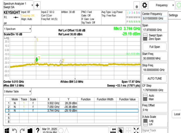
Band77-Part27_50MHz_DFT_s_OFDM_SCS30kHz_BPSK_RB1_1_CH635000_below 18G
