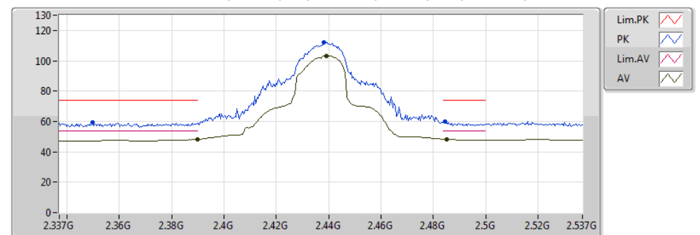
RE above 1GHz;Band:2.4G;HT20;BWch:20MHz;Nss:1,(M0);Nant:2;Ch:2437MHz;TX
