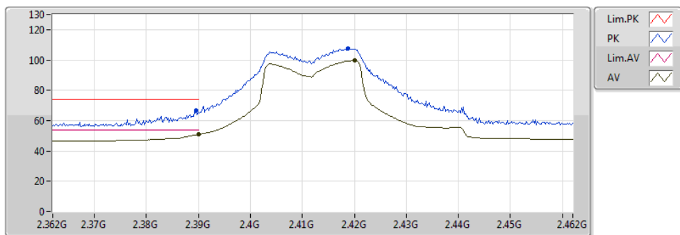
RE above 1GHz;Band:2.4G;HT20;BWch:20MHz;Nss:1,(M0);Nant:2;Ch:2412MHz;TX
